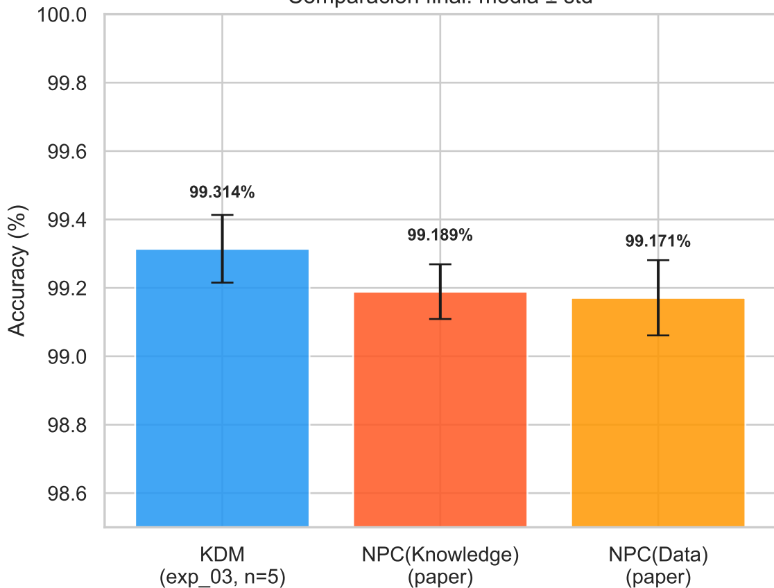
Comparación final: media \pm std
