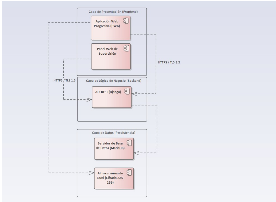
Figura 2.7: Diagrama de Componentes (Arquitectura en 3 Capas)
