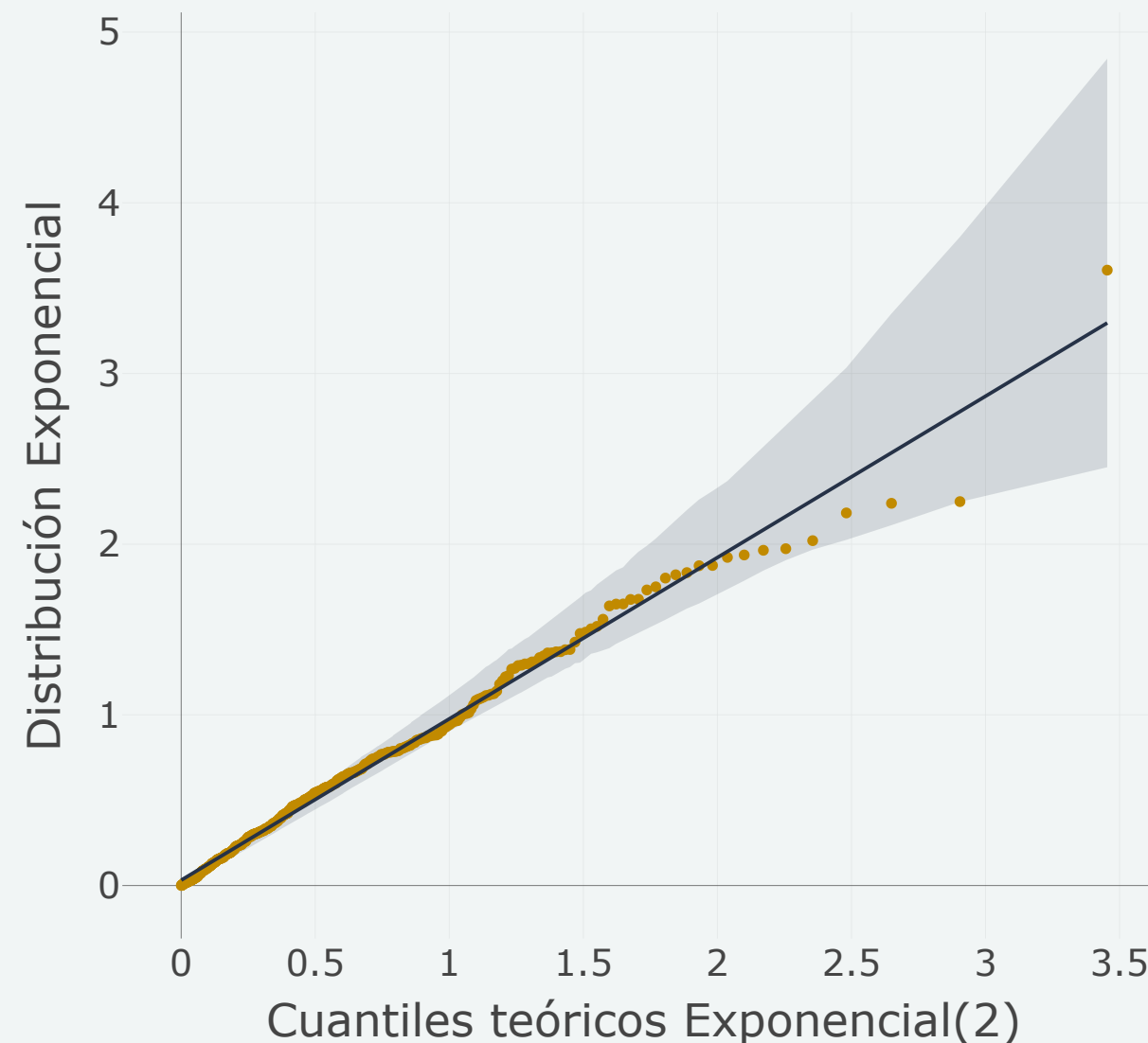
QQ-plot (exponencial)
