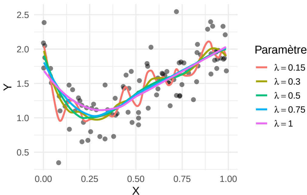
Figure 2: Différents estimateurs de la fonction f .
