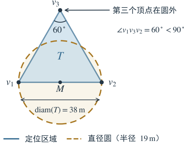
图 2 等边三角形的直径圆无法覆盖整个定位区域。三角形边长为 38 米，以边 v_1v_2 为直径的圆半径为 19 米，第三个顶点 v_3 位于圆外
