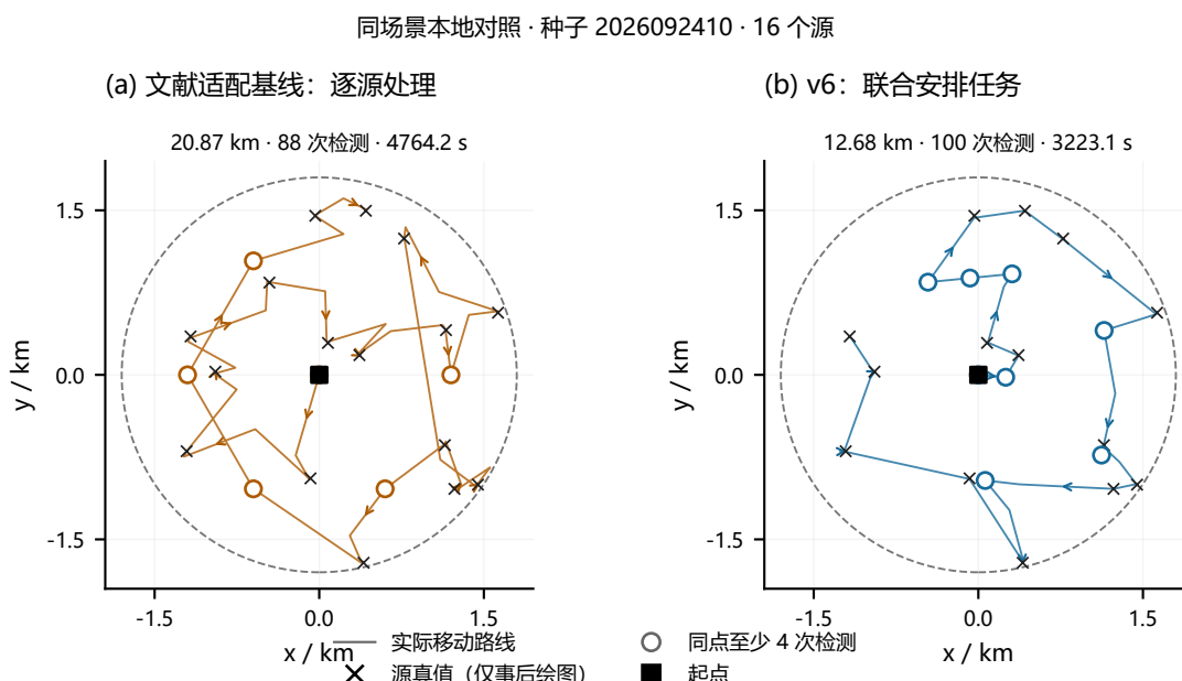
图 10 同一场景的本地路线对照（种子 2026092410）。坐标、比例与源真值相同，连线来自实际动作，箭头示方向；圆点为至少执行四次检测的位置。真值只用于事后绘图，不输入策略。
