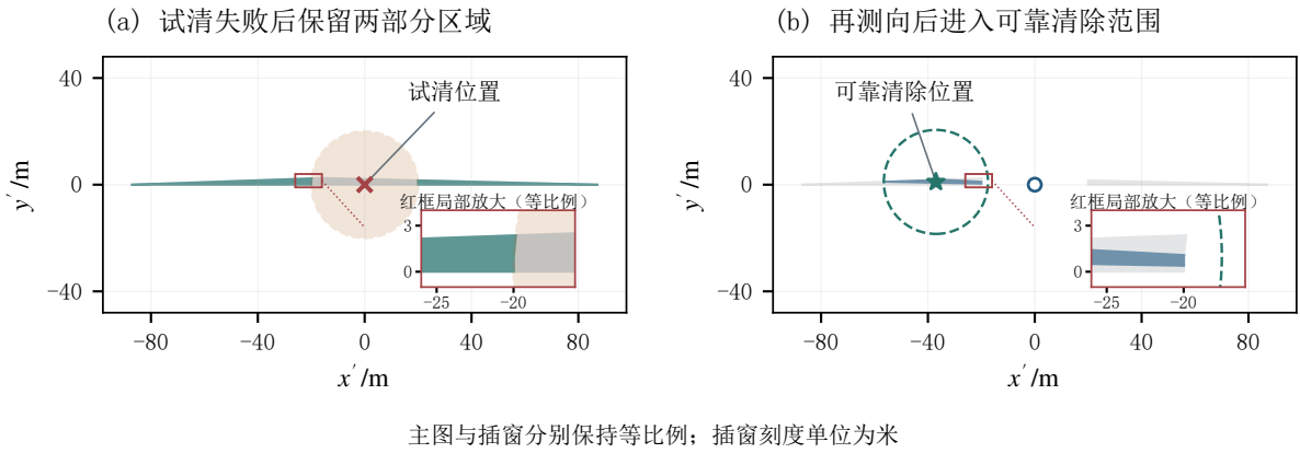
图 8 实际试清失败与后续定位。主图保持等比例，插图为明确标注的局部放大。蓝色表示观测位置域，绿色表示试清失败后保留部分，灰色为后续测向前区域；圆圈分别为 20 米试清和 19.5 米可靠清除范围。局部坐标仅由平移、旋转得到，未使用真实源坐标。
