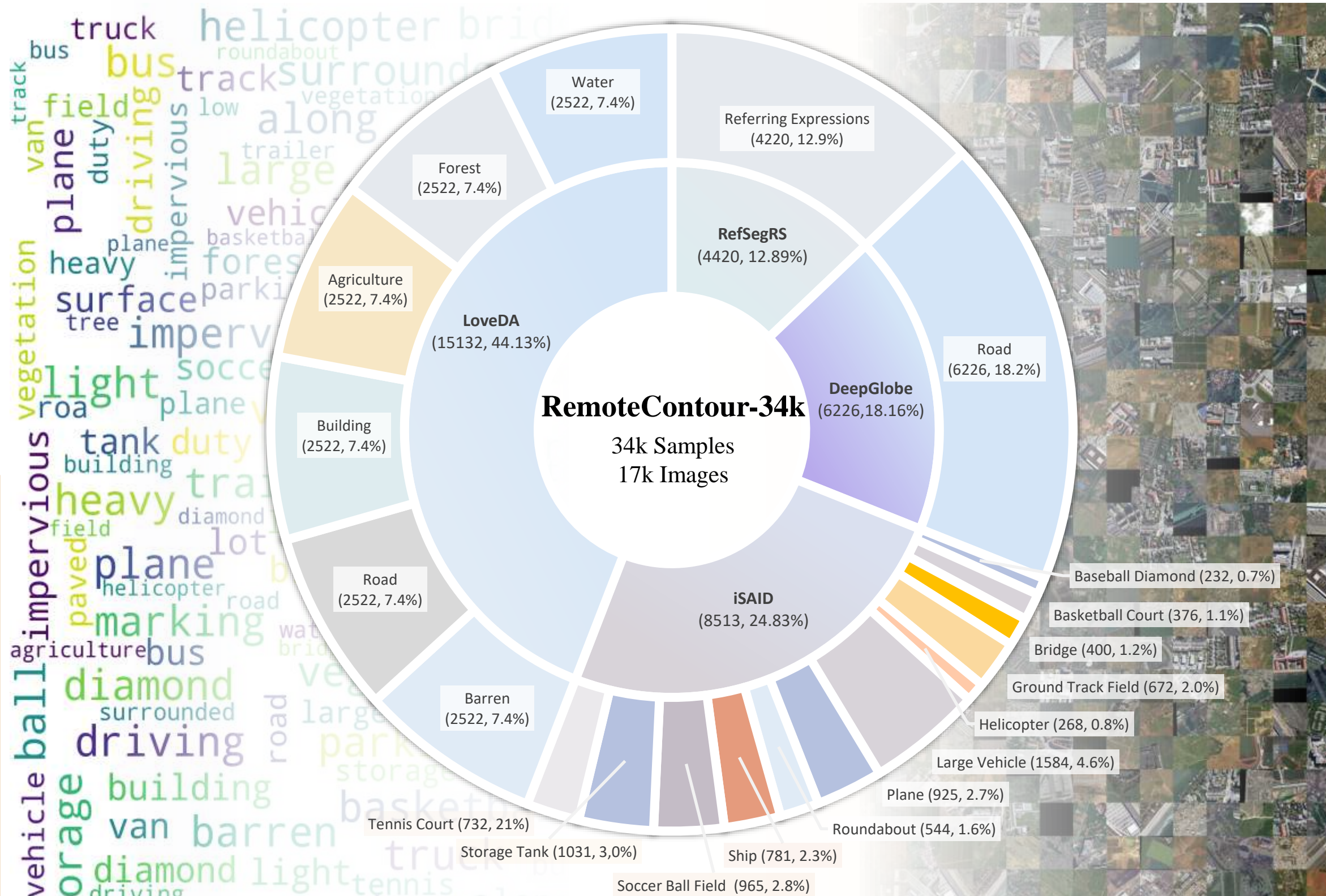
LoveDA
