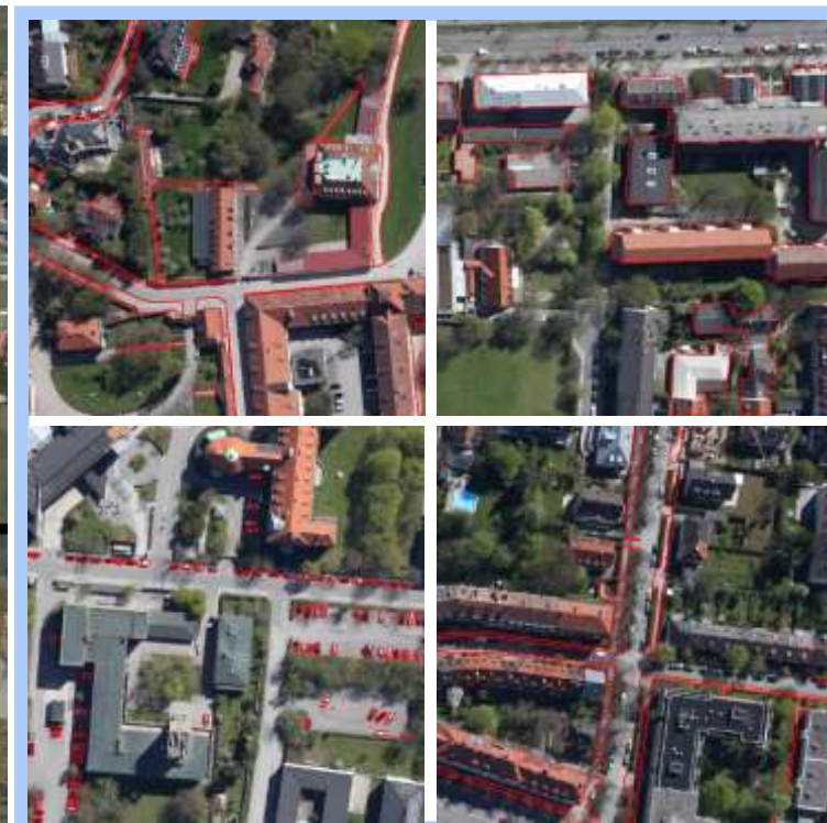
LoveDA
