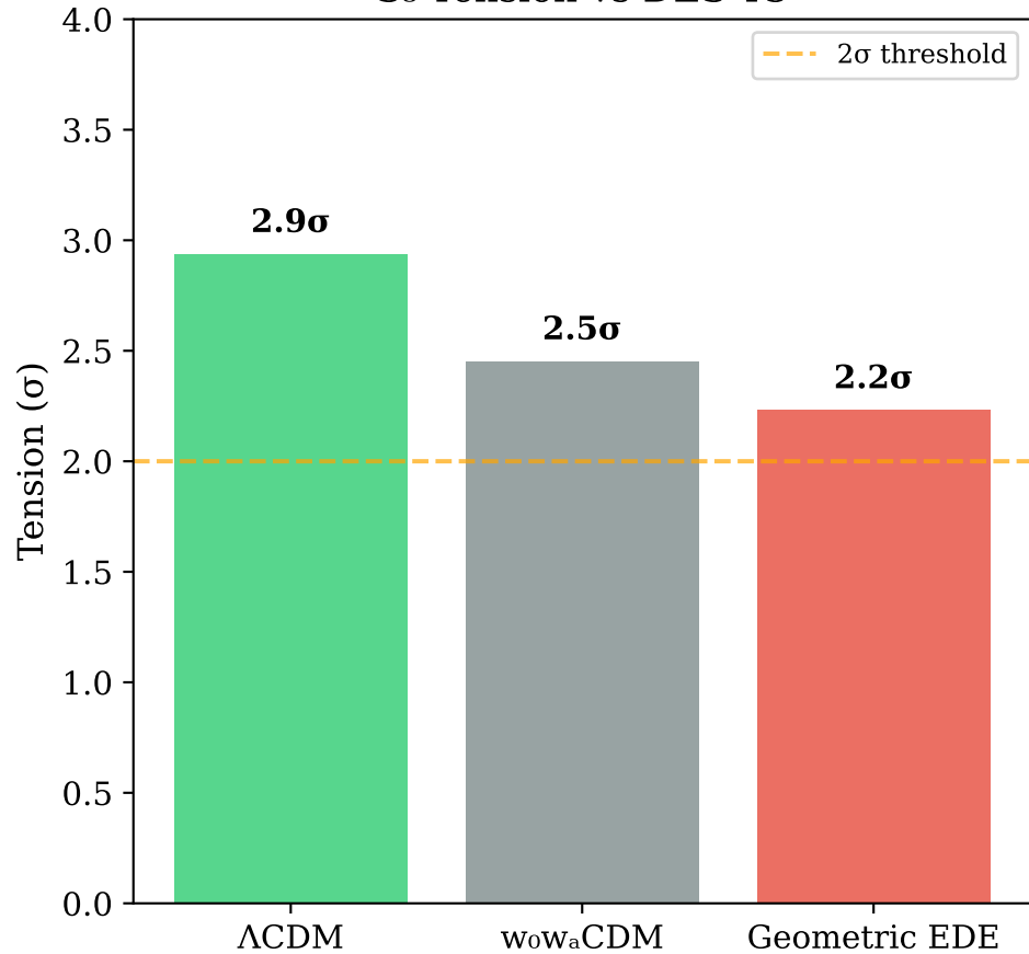
S 8 Tension vs DES Y3
