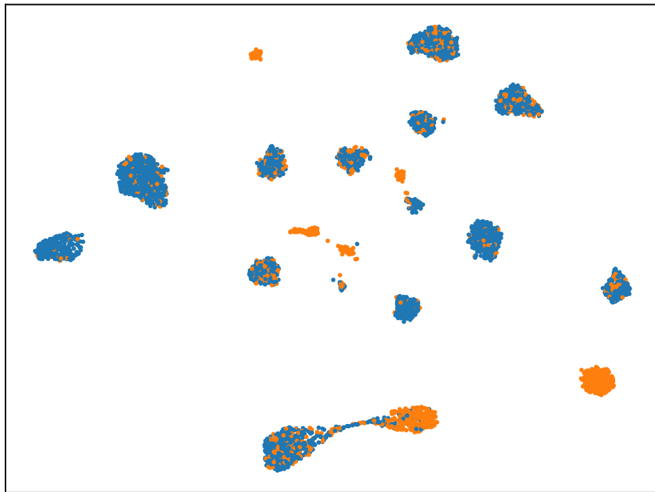
giniclust3
