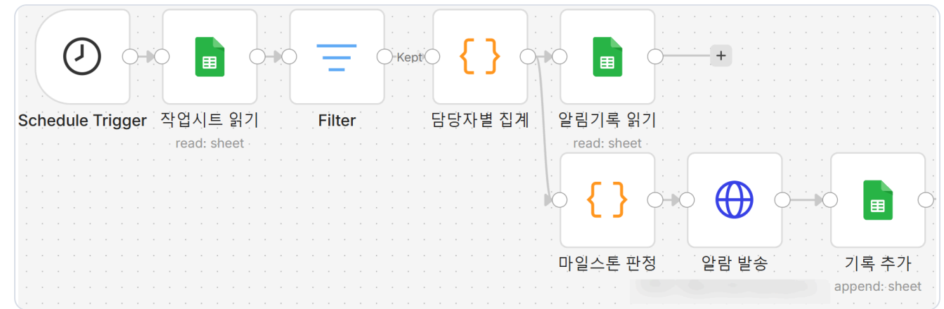
작업 시트 조회부터 담당자별 집계, 알림 발송과 이력 기록까지 연결한 n8n 워크플로우
