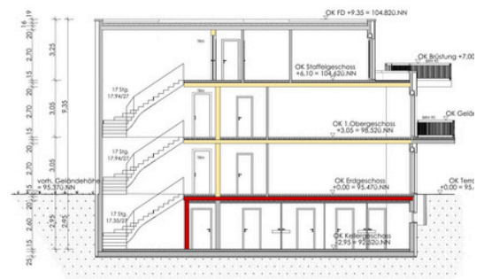
SNITT Schnitt A-A Haus 2
