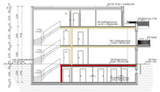
SCHNITT Schnitt A-A Haus 2
