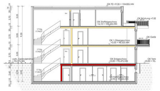
Schnitt A-A Haus 2
