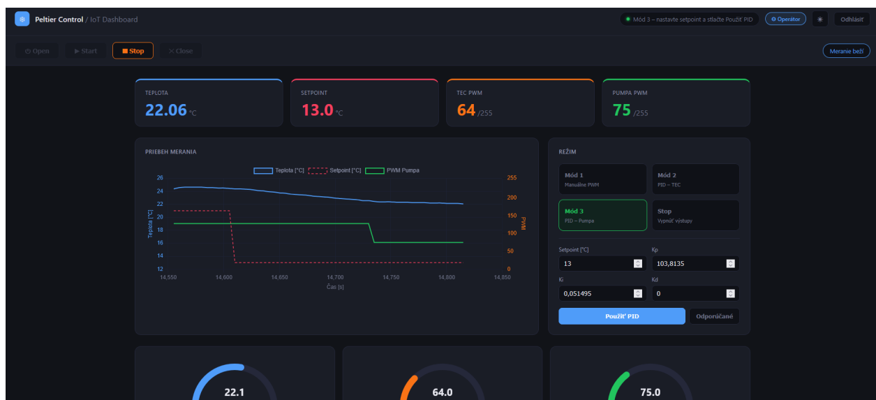
Obr. 15: Dashboard v Móde 3 (PID – Pumpa) – regulácia prietoku pumpy
