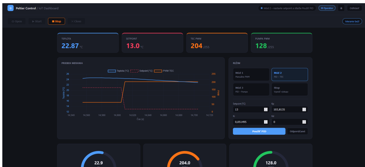
Obr. 14: Dashboard v Móde 2 (PID – TEC) – regulácia TEC PWM s viditeľným skokom setpointu
