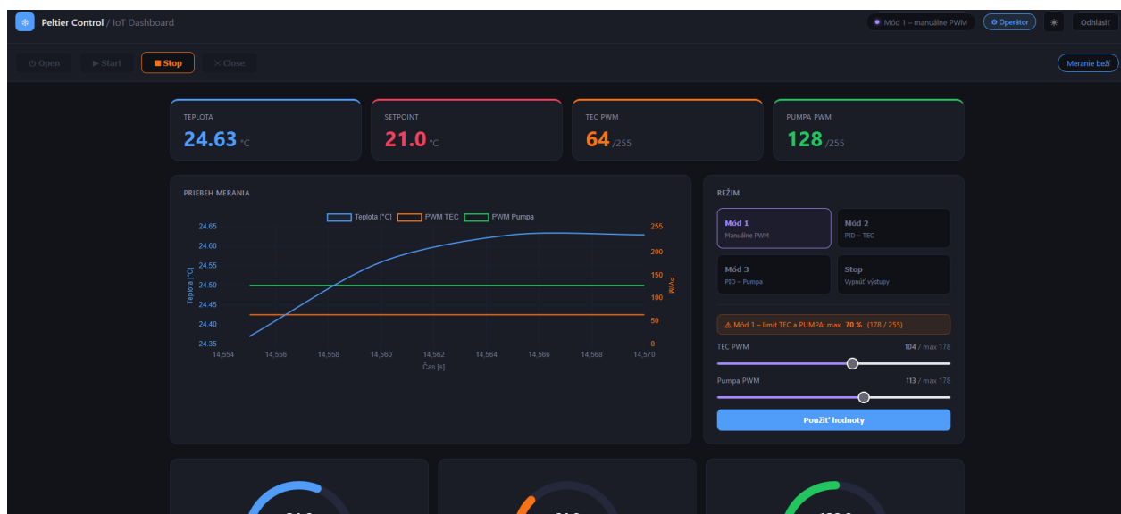
Obr. 15: Dashboard v Móde 1 (manuálne PWM) – priebeh merania s grafom teploty a PWM
