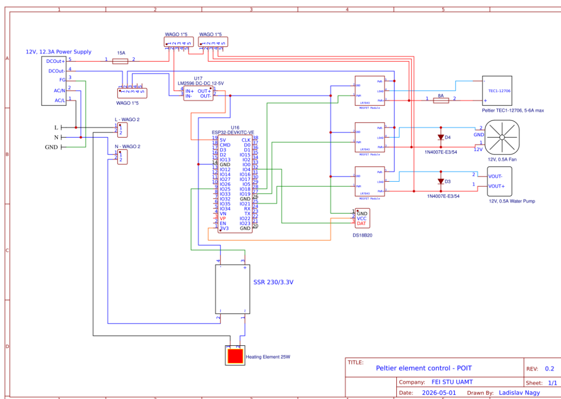
Obr. 1: Schéma zapojenia hardvérových komponentov systému
