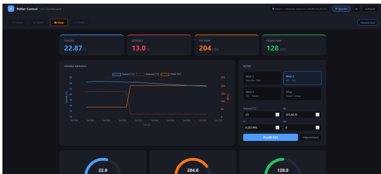
Obr. 16: Dashboard v Móde 2 (PID – TEC) – regulácia TEC PWM s viditeľným skokom setpointu
