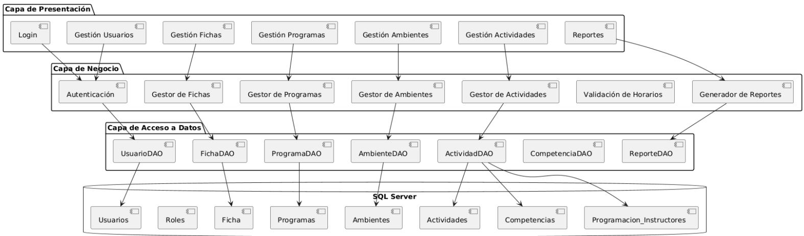
Arquitectura N-Tier - Sistema ClassControl
