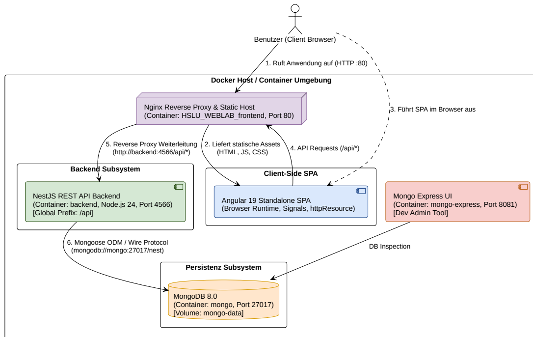
Figure 2: Bausteinsicht Level 1: System-Whitebox mit Containern und Ports (PlantUML: 02_bausteinsicht_level1.puml)
