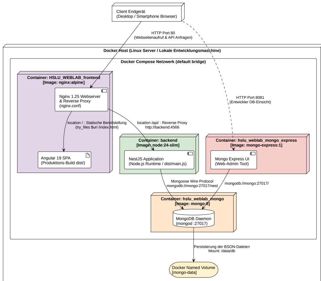
Figure 8: Verteilungssicht: Docker Compose Umgebung (PlantUML: 08_verteilungssicht_deployment.puml)
