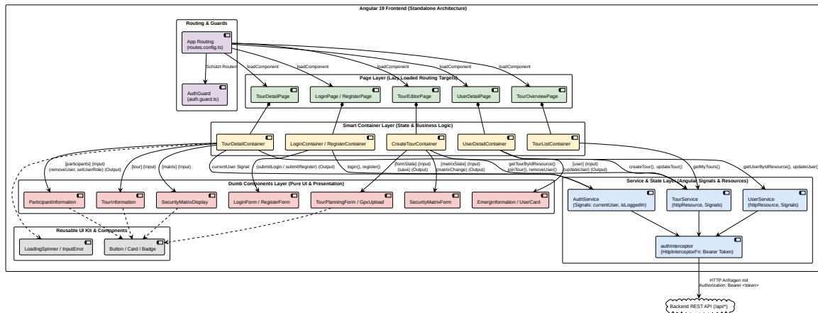
Figure 3: Bausteinsicht Level 2: Frontend-Aufbau mit Smart Containern und Dumb Components (PlantUML: 03_frontend_architektur.puml)
