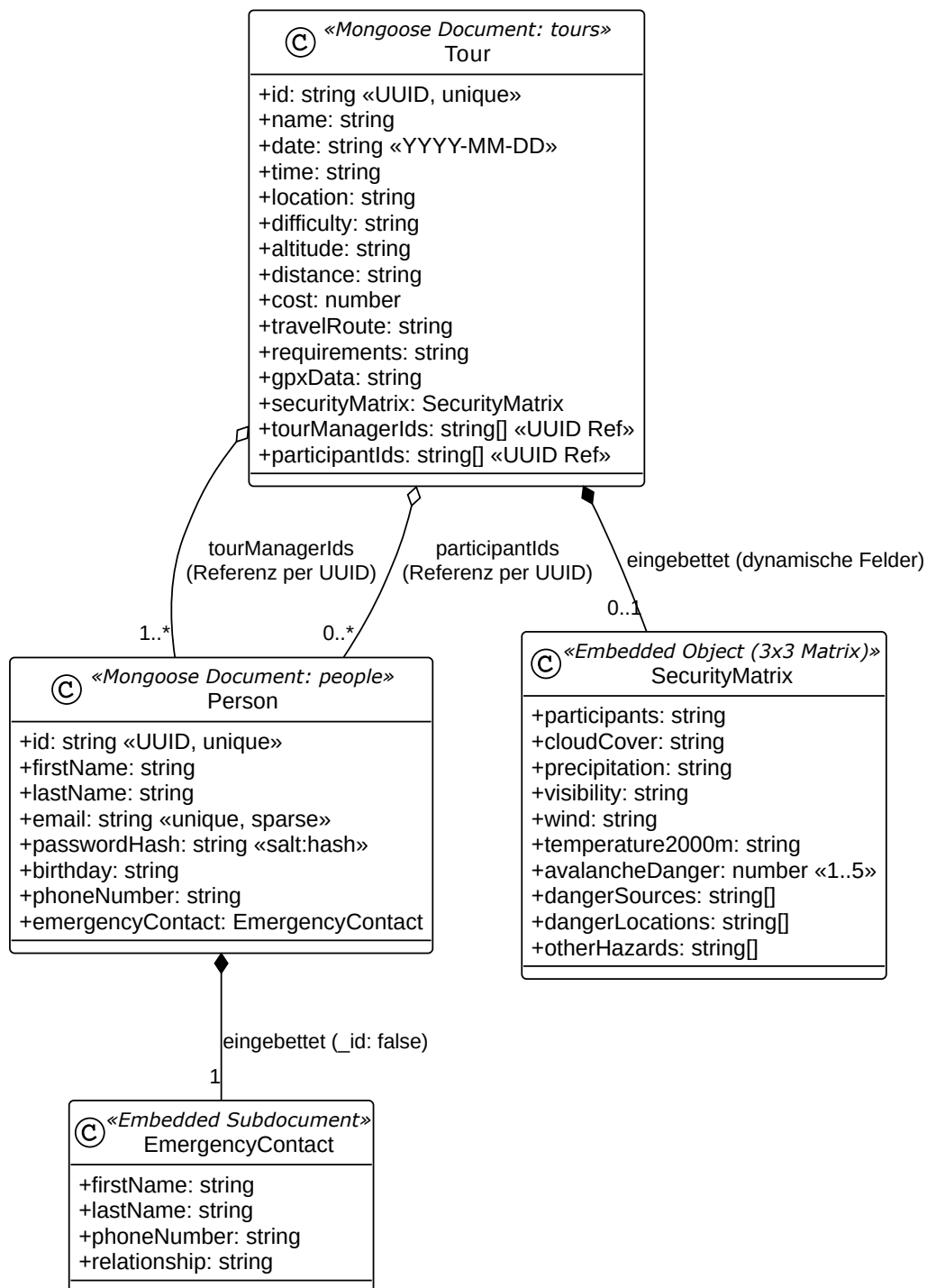
Figure 9: Datenmodell: Mongoose Schemas und Beziehungen (PlantUML: 09_datenmodell_persistenz.puml)
