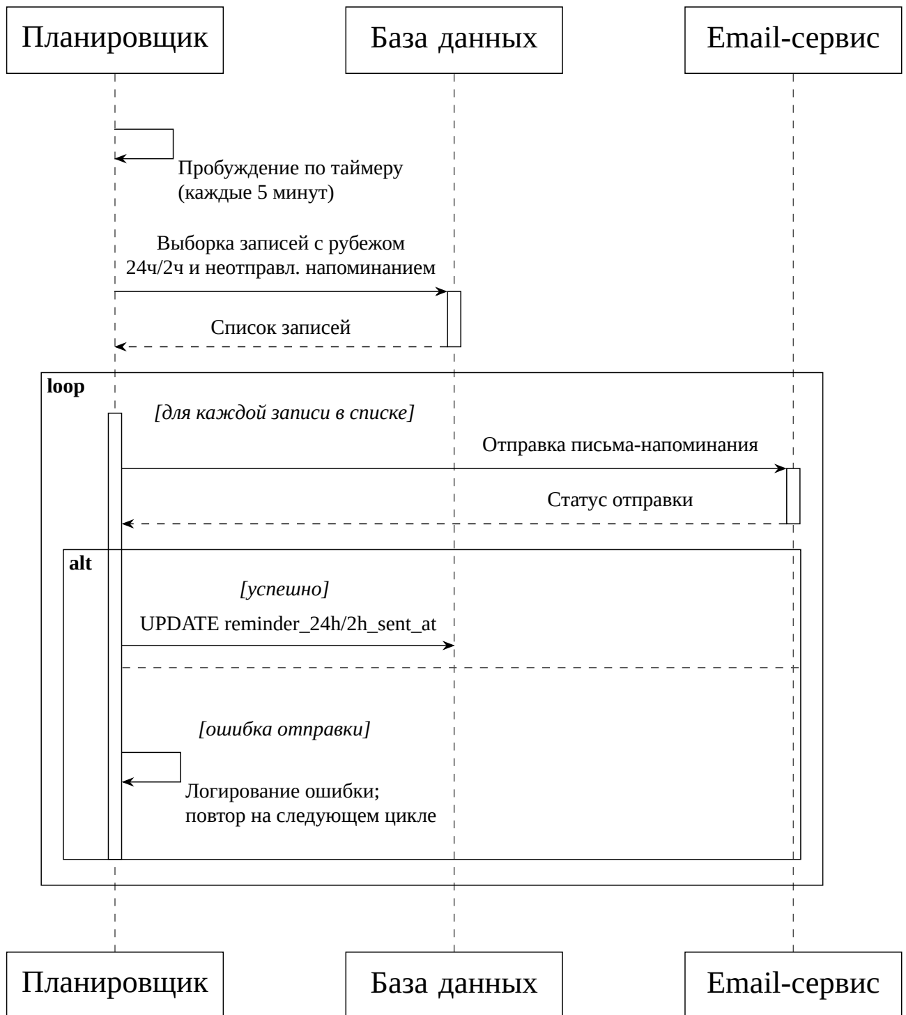
Рисунок Б.5 – Диаграмма последовательностей бизнес-процесса «Автоматическая отправка напоминаний» (FR-008)
