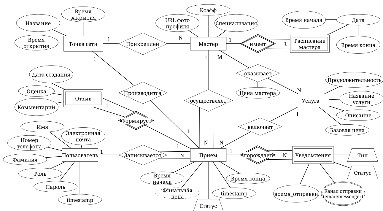
Рисунок 1 – Инфологическая модель – бизнес-домен
