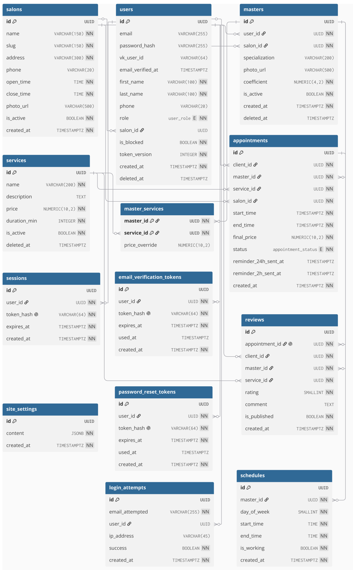
Рисунок 4 – Дatalogическая модель – физическая схема БД
