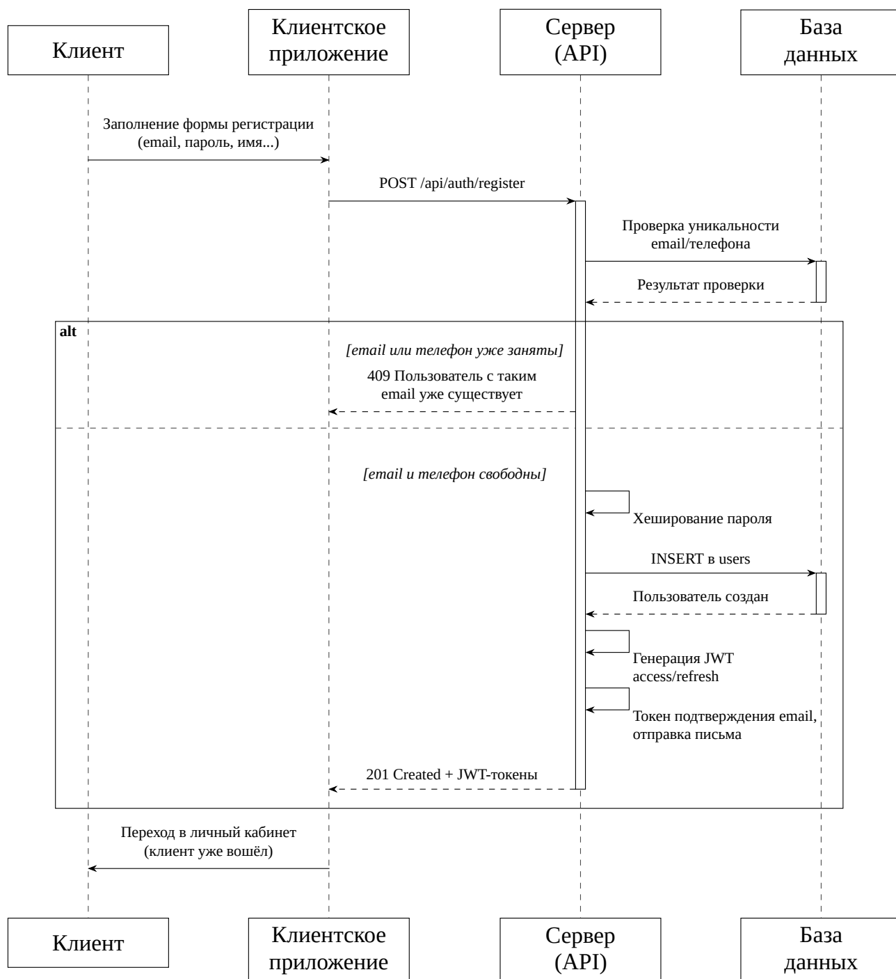
Рисунок А.1 – Диаграмма последовательностей бизнес-процесса «Регистрация» (ФТ-001)
