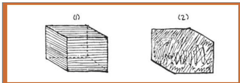
Figura 5: Construcción del cubo a partir de planos superpuestos, según la explicación de la esfera.
