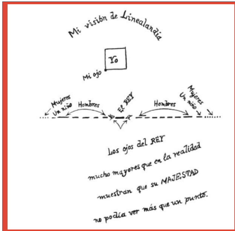
Figura 1: Representación de la visión de Cuadrado en Linealandia.
