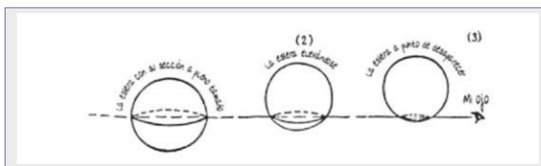
Figura 3: Secciones de una esfera al atravesar el plano de Planilandia.
