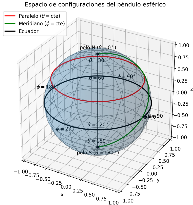
Figura 2: Espacio de configuraciones del péndulo esférico Q : cada punto de la superficie esférica representa una orientación posible de la varilla de longitud l , parametrizada por los ángulos \theta (inclinación) y \phi (azimutal).
