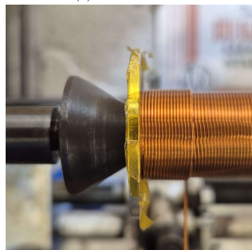
(d) Exemplar coil end
