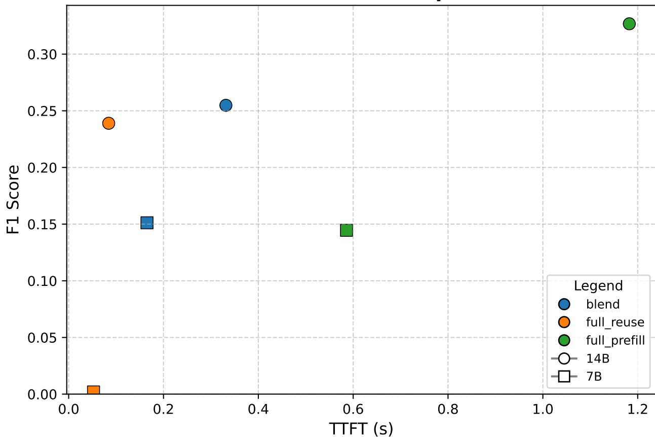
Dataset: wikimqa
