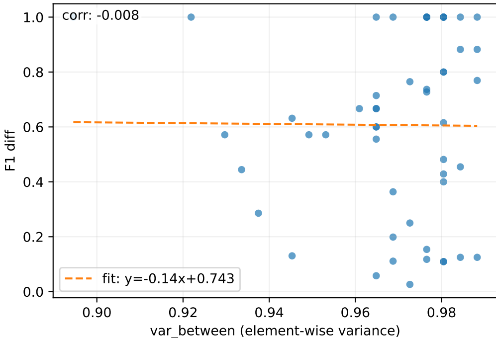
blend vs full prefill — F1
