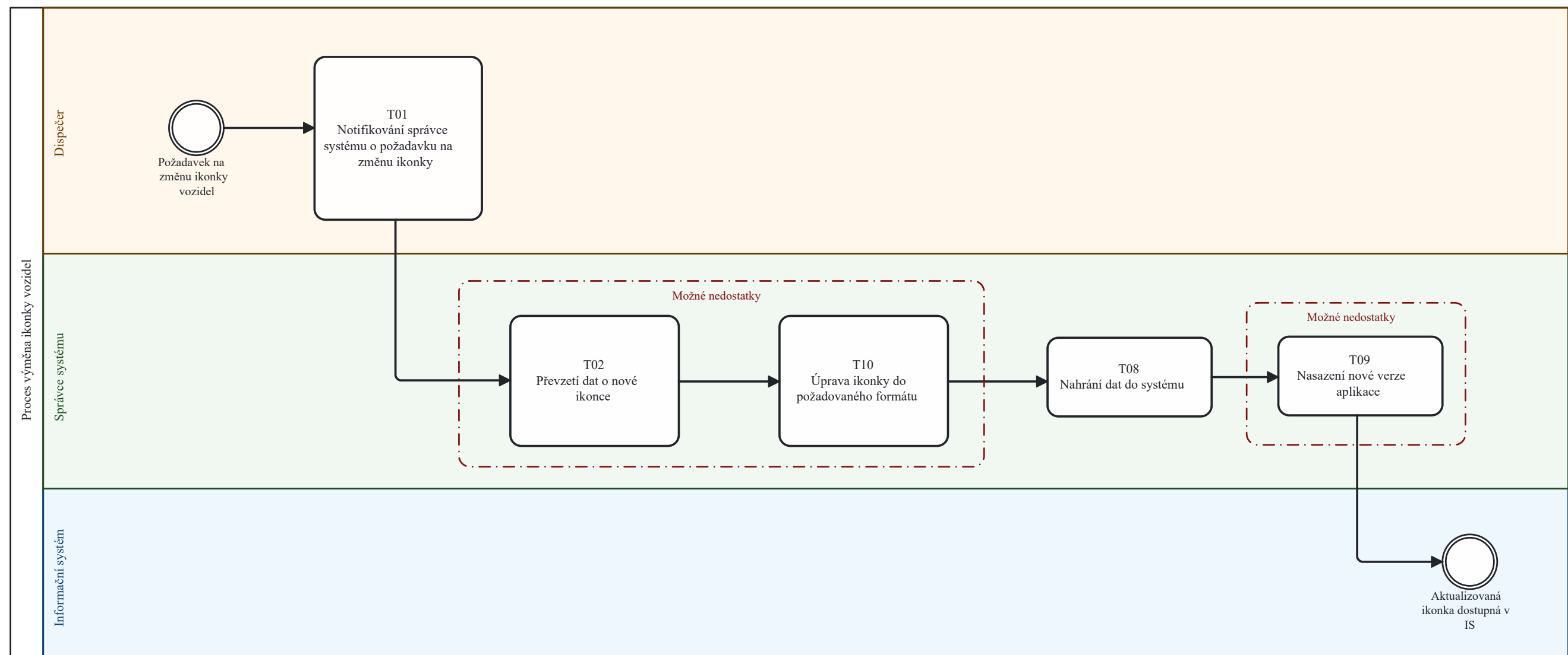
Obrázek 8: BPMN diagram Pr3 Výměna ikonky vozidel
