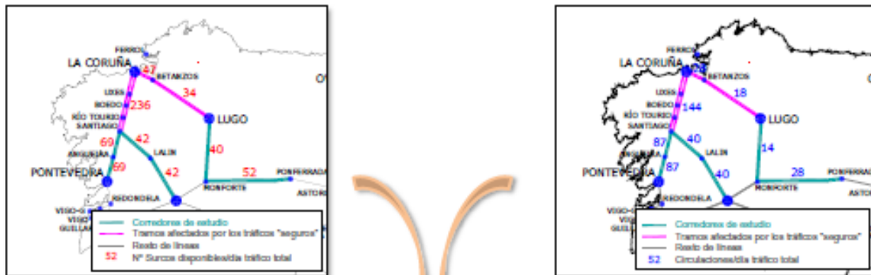
CAPACIDAD DIARIA ACTUAL TRÁFICO TOTAL (VIAJEROS + MERCANCIAS) (2012)
