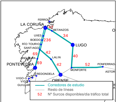
CAPACIDAD DIARIA ACTUAL TRÁFICO TOTAL (VIAJEROS + MERCANCÍAS) (2012)
