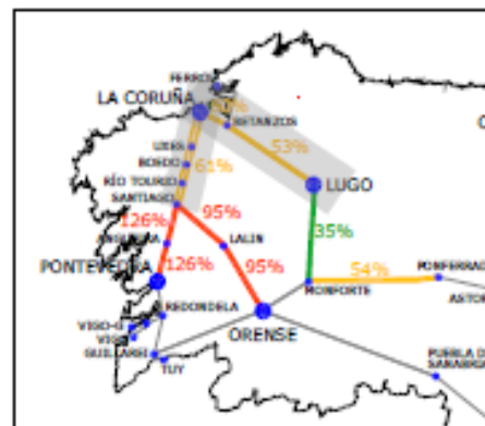
GRADO DE OCUPACIÓN TRÁFICO TOTAL (ACTUAL + TRÁFICOS SEGUROS) (2017)
