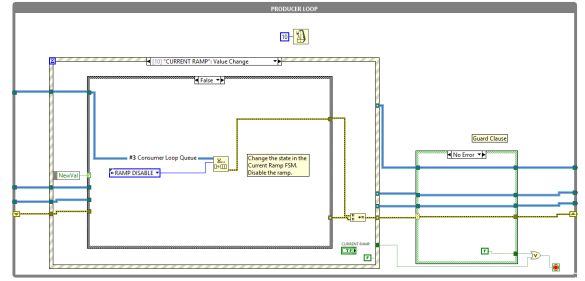
(d) RAMP DISABLE state
