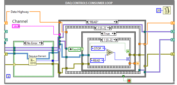
(d) DAQ Controls Consumer Loop: READ state, frame 2 (II)
