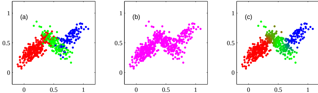
图 9.5 从图 2.23 所示的由 3 个高斯分布组成的混合模型中抽取的 500 个点的示例。(a) 来自联合分布 p(\mathbf{z})p(\mathbf{x} | \mathbf{z}) 的样本，其中变量 z 的三个状态（对应于混合模型的三个分量）分别用红色、绿色和蓝色表示；(b) 来自边缘分布 p(\mathbf{x}) 的相应样本，该分布是通过简单地忽略 \mathbf{z} 的取值、仅绘制 \mathbf{x} 的取值而得到的。(a) 中的数据集被称为“完整的”，而 (b) 中的数据集则是“不完整的”。(c) 相同的一组样本，其中颜色表示与数据点 \mathbf{x}_n 相关的责任度 \gamma(z_{nk}) 的取值，通过按比例使用红色、蓝色和绿色墨水来绘制对应的数据点，这些比例分别由 k = 1, 2, 3 时的 \gamma(z_{nk}) 给出。
