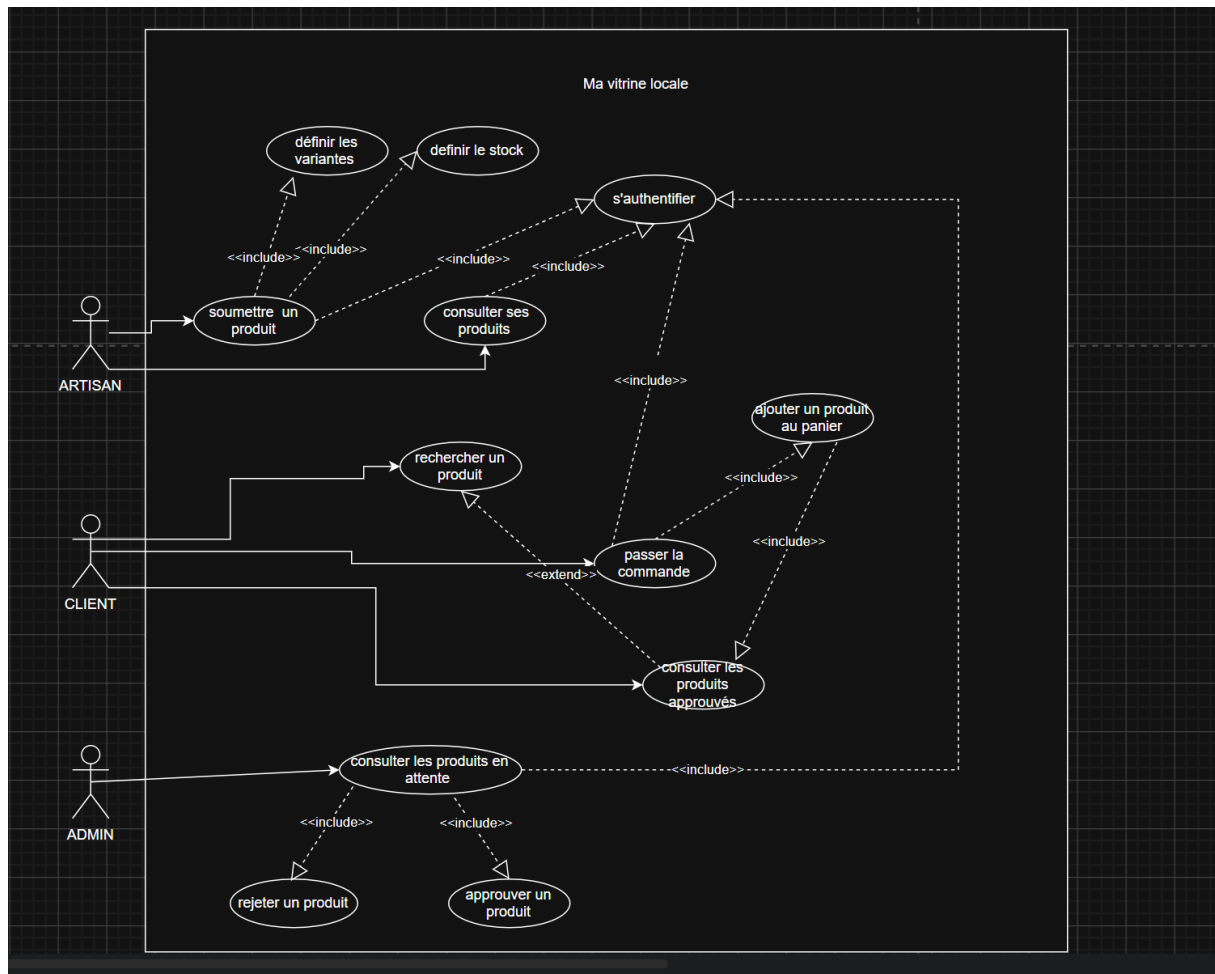
Diagramme du cas d'utilisation
