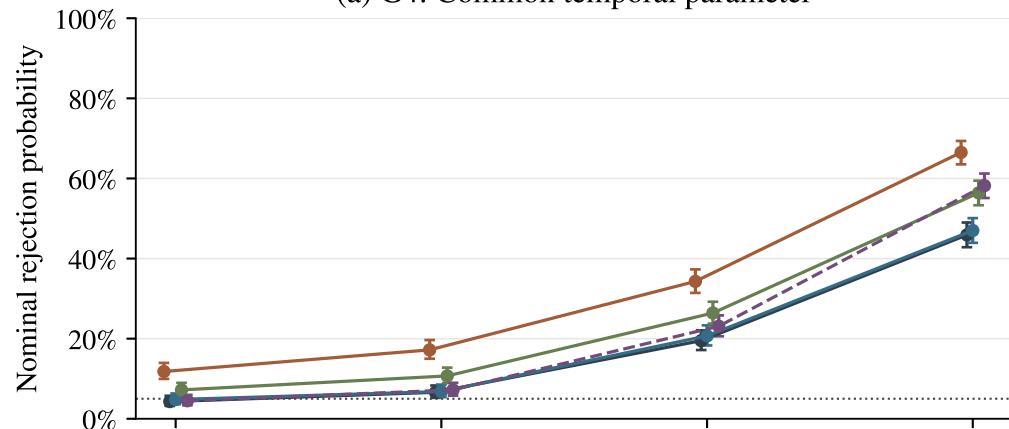
(a) G4: Common temporal parameter
