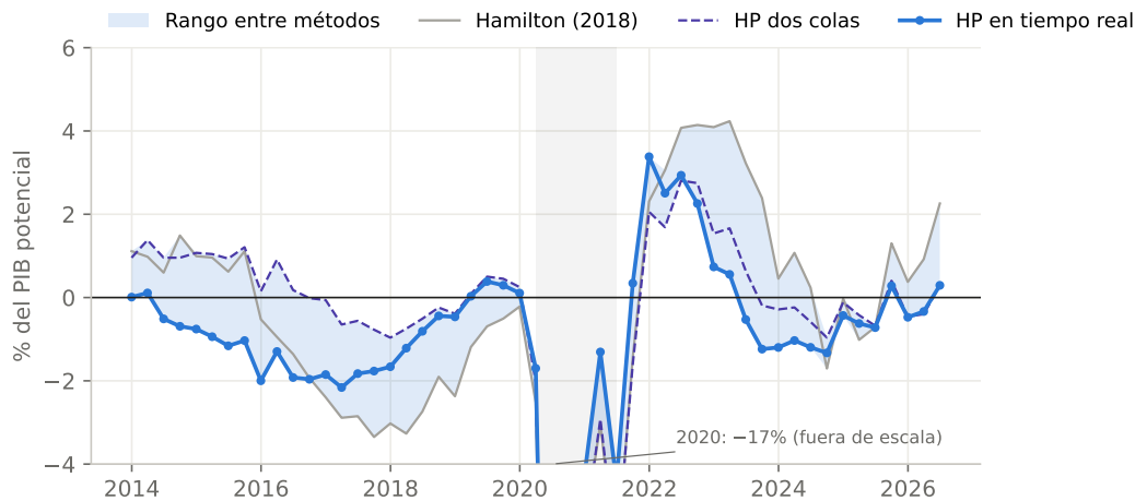
Figura 16: Brecha del producto con los tres métodos (figura vectorial).
