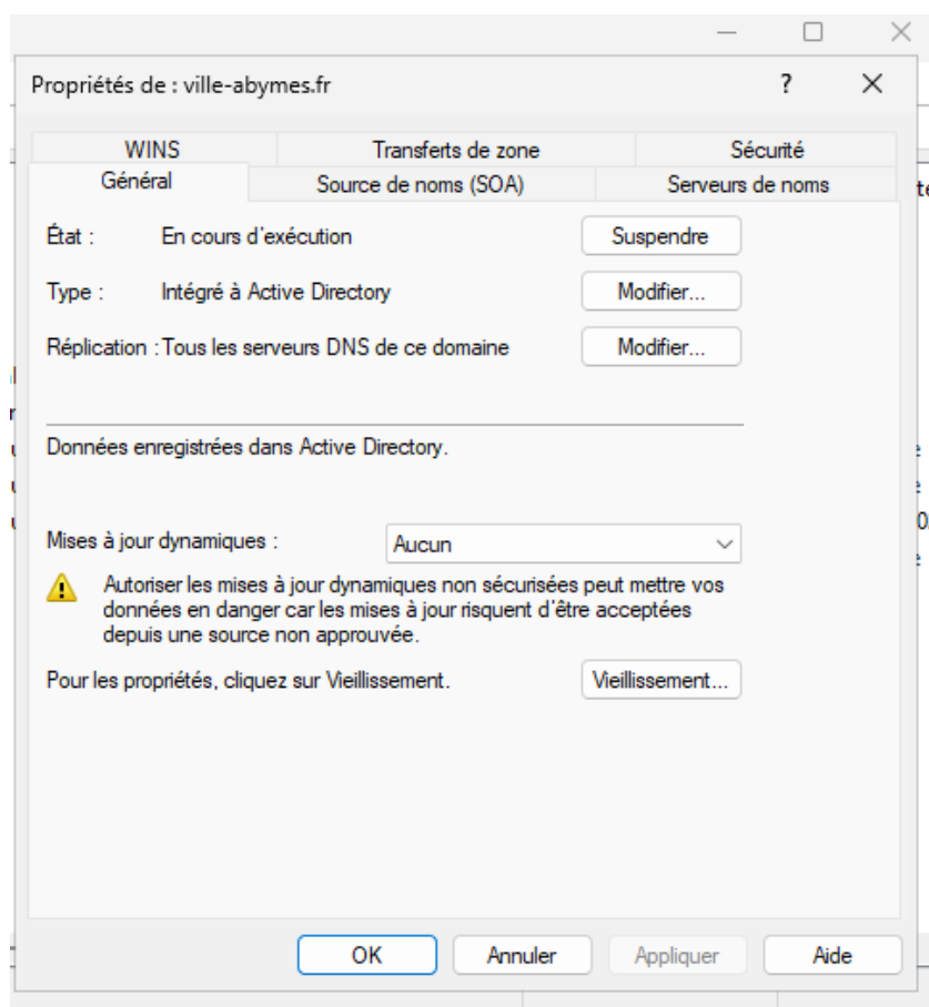
Figure 22 — Propriétés de la zone de recherche directe ville-abymes.fr
