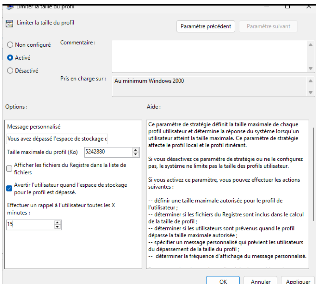
Figure 82 — Limitation de la taille des profils itinérants à 5 Go
