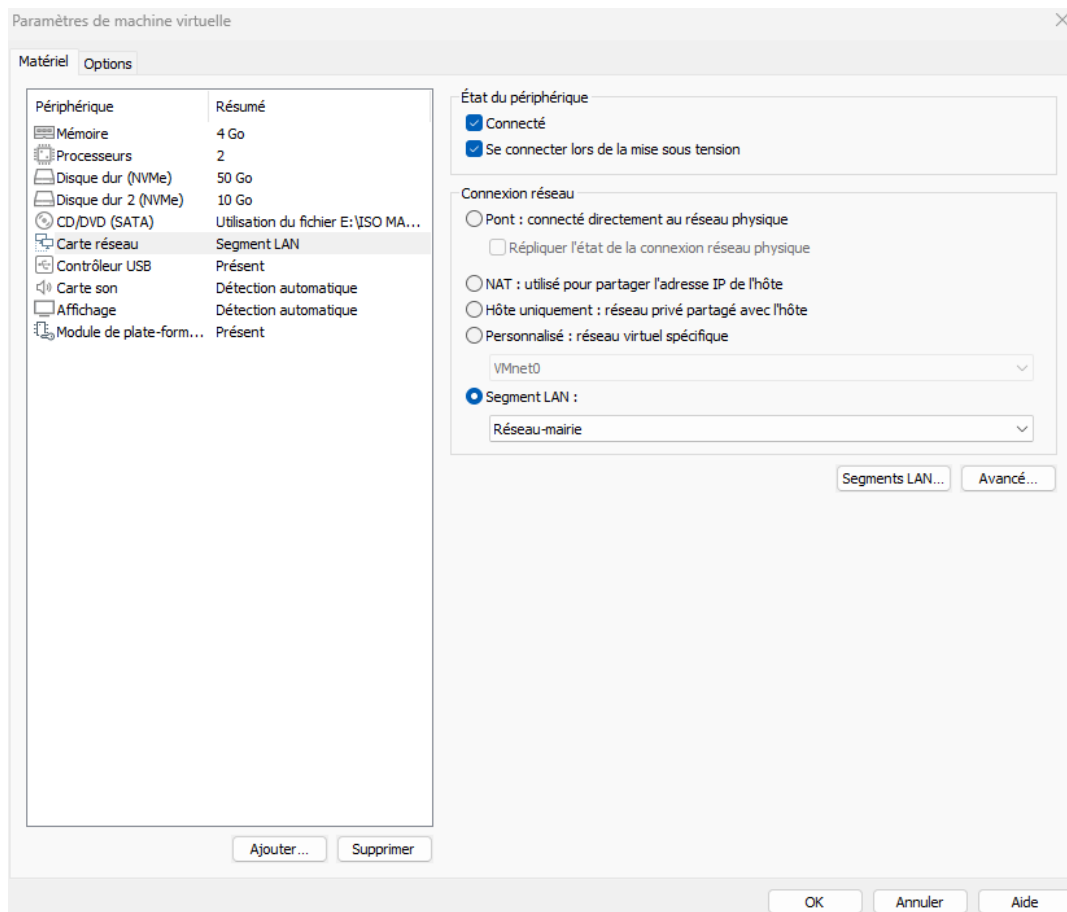
Figure 9 — Paramètres matériels définitifs de srvad et mode réseau
