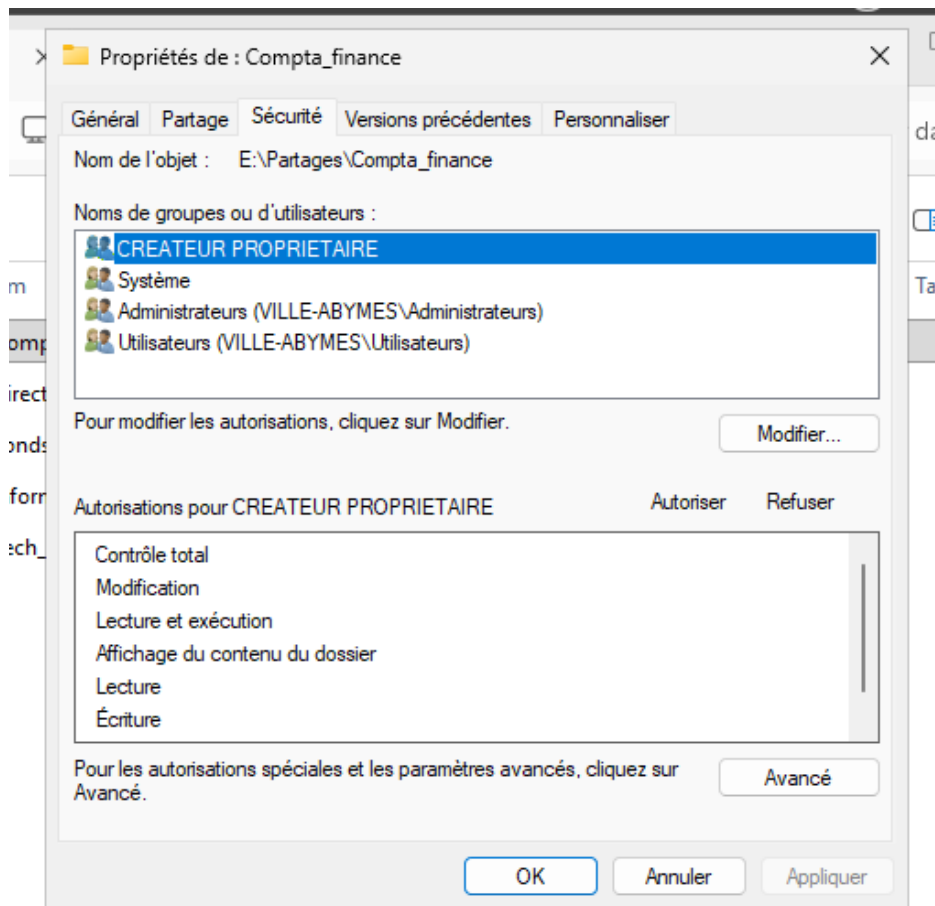
Figure 66 — Autorisations NTFS du dossier E:\Partages\Compta_finance
