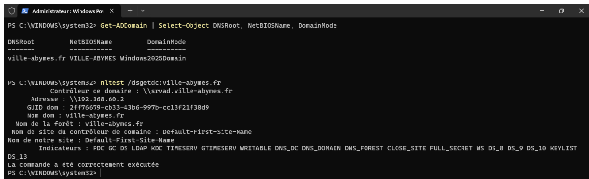
Figure 20 — Vérification de la promotion en contrôleur de domaine
