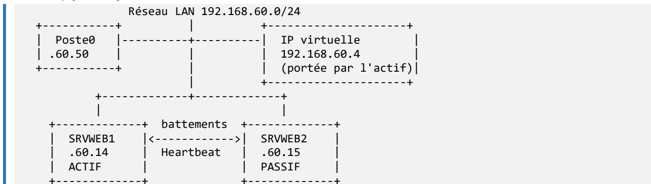
Schéma simplifié de l'infrastructure
