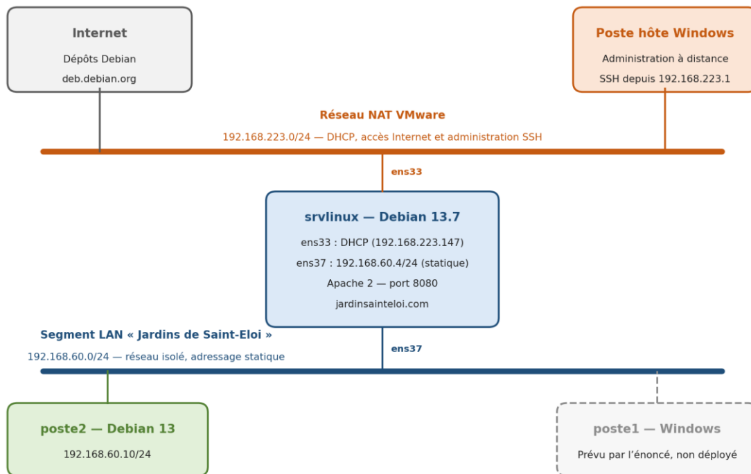
Schéma 1 – Architecture réseau réalisée
