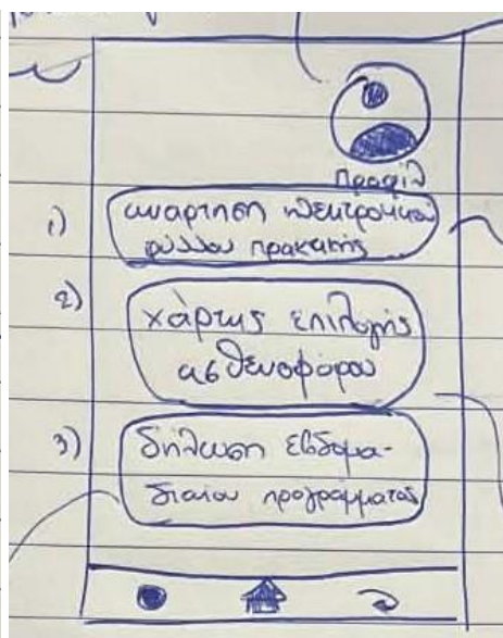
Σελίδα Σπουδαστή
