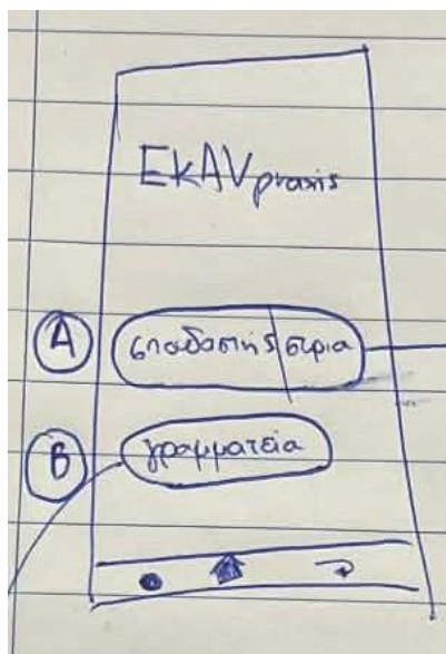
Αρχική Σελίδα
