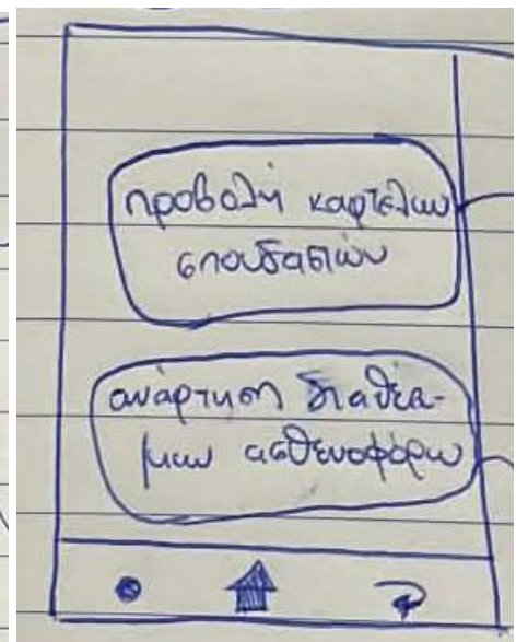
Σελίδα Γραμματείας
