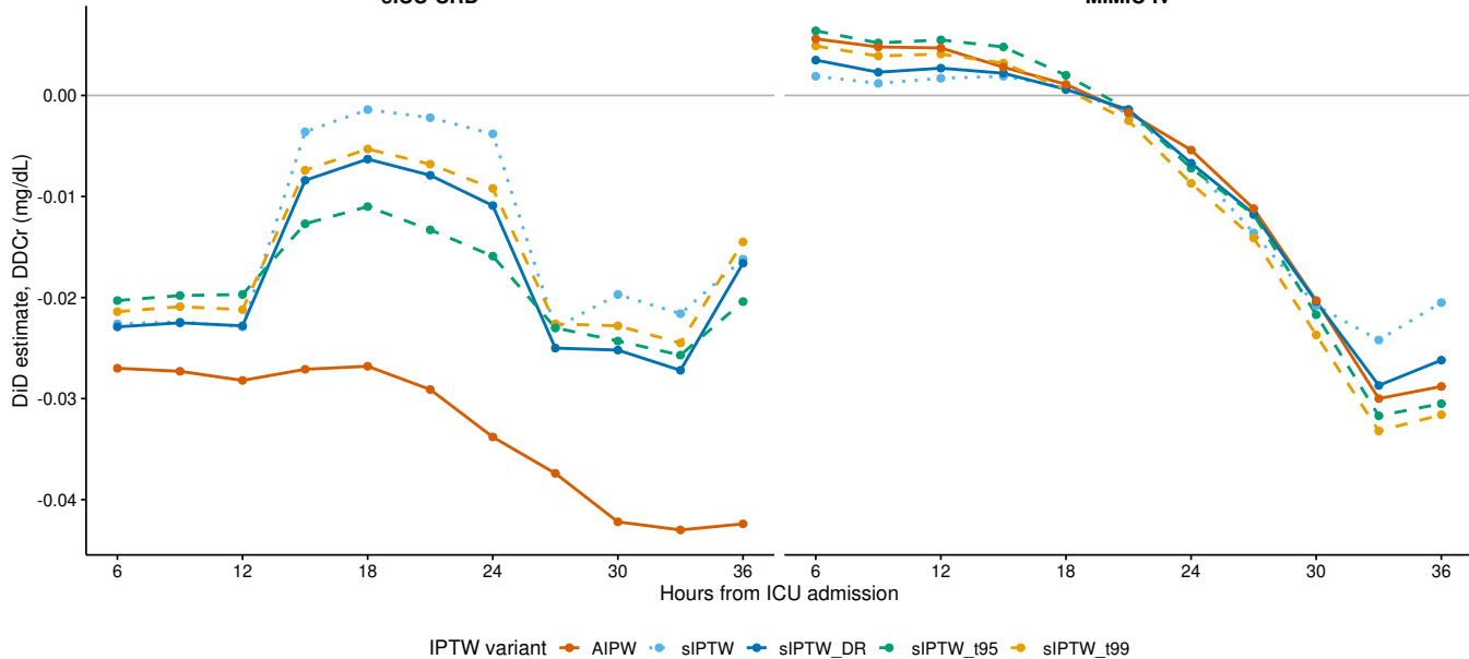
eICU-CRD
