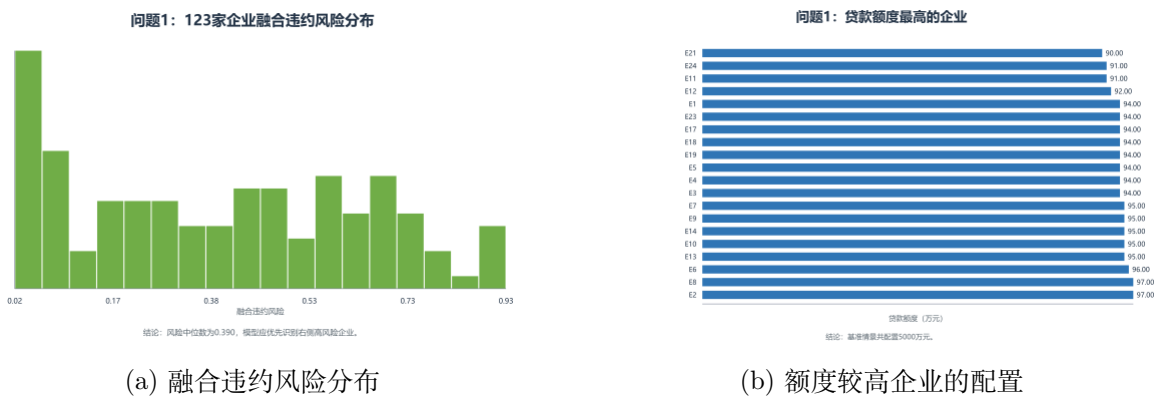
图 6-1 问题一风险与信贷配置结果
