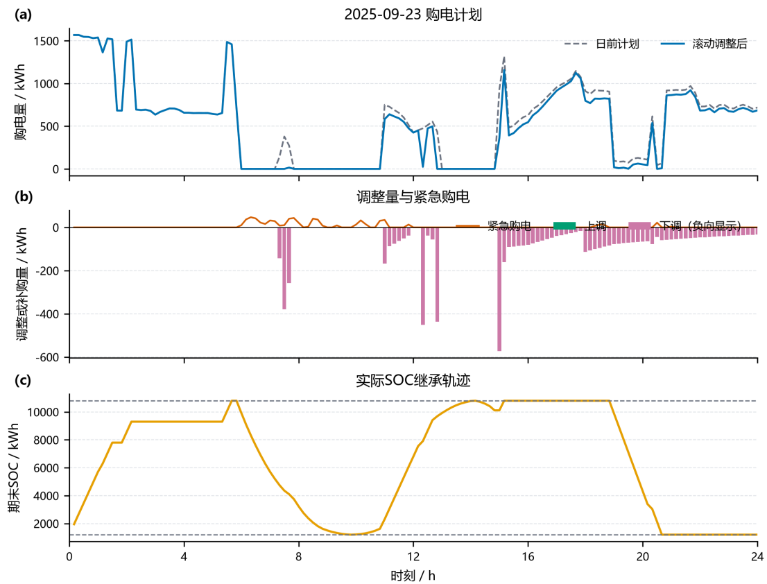
图 14 日前计划与四时点滚动调整的典型日对比
