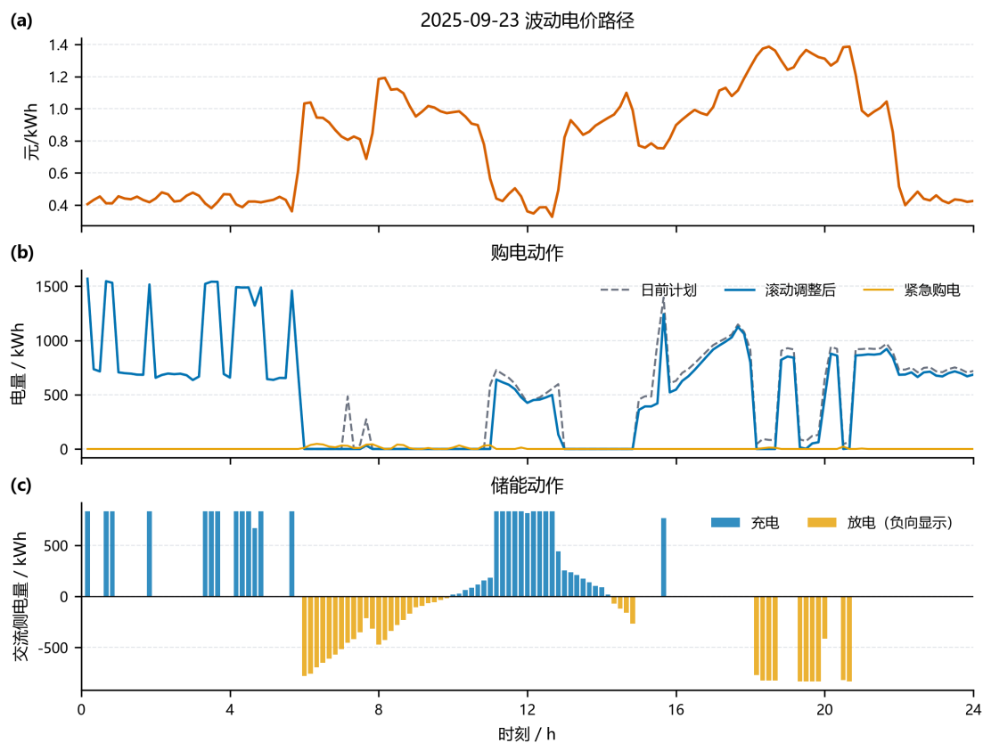
图 19 波动电价下滚动策略的典型日调度
