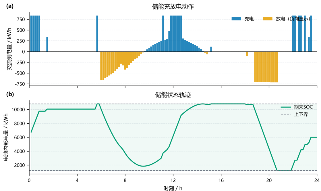
图 5 问题一储能状态与充放电行为
