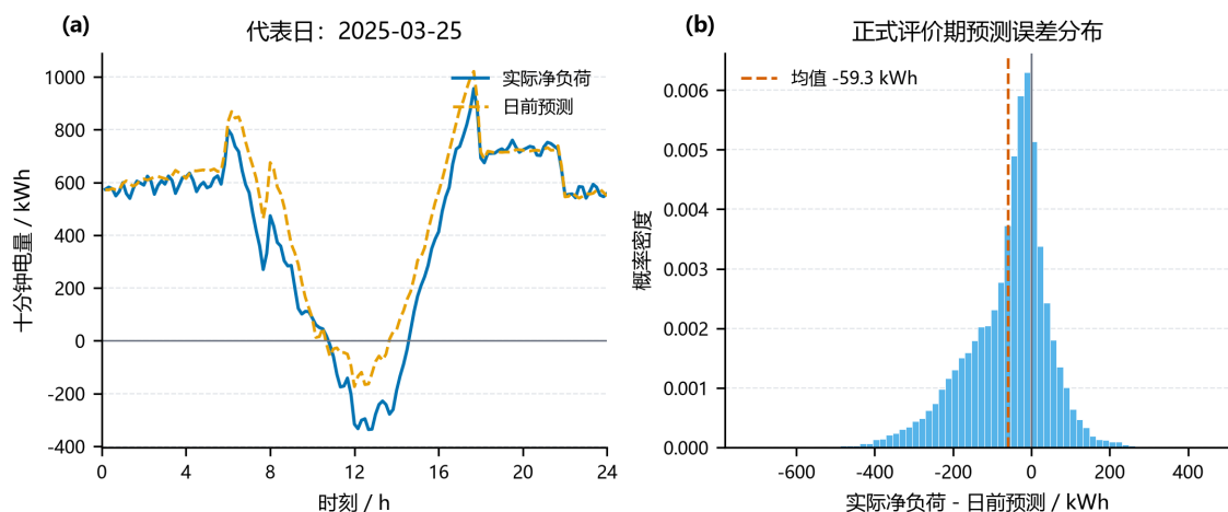
图 9 实际净负荷与日前预测误差
