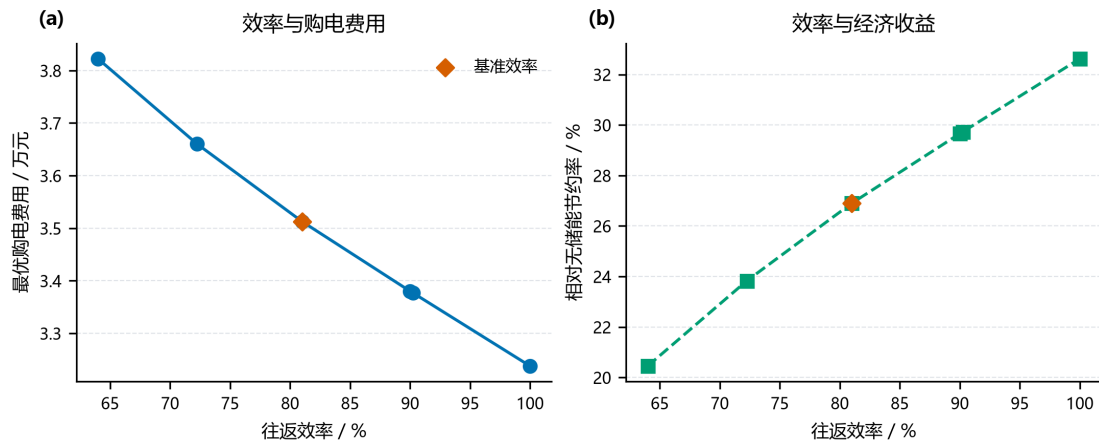
图 7 问题一储能效率敏感性
