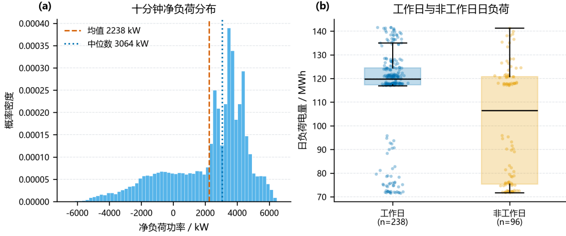
图 2 净负荷分布与工作日差异
