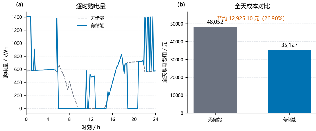
图 6 问题一有无储能购电策略对比
