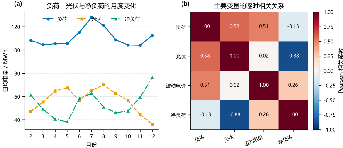
图 3 主要变量月度变化与相关关系
