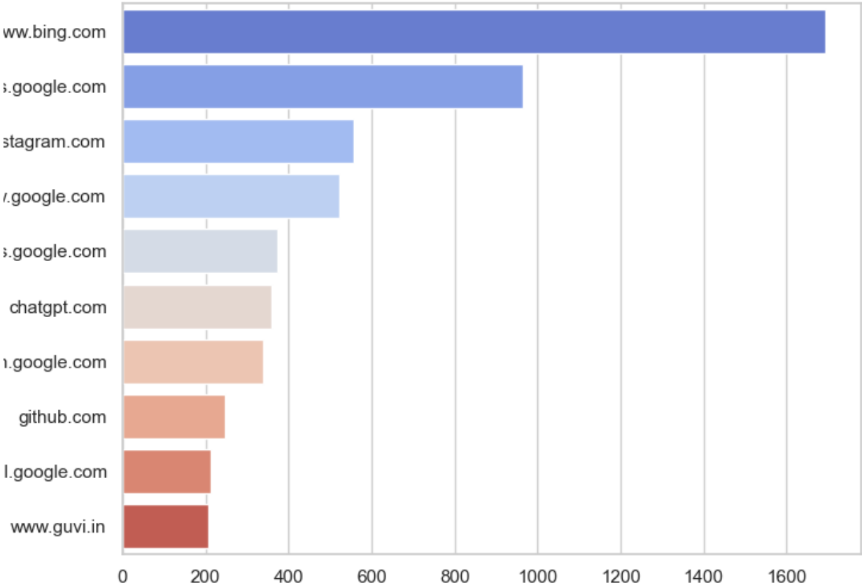
Top Domains
