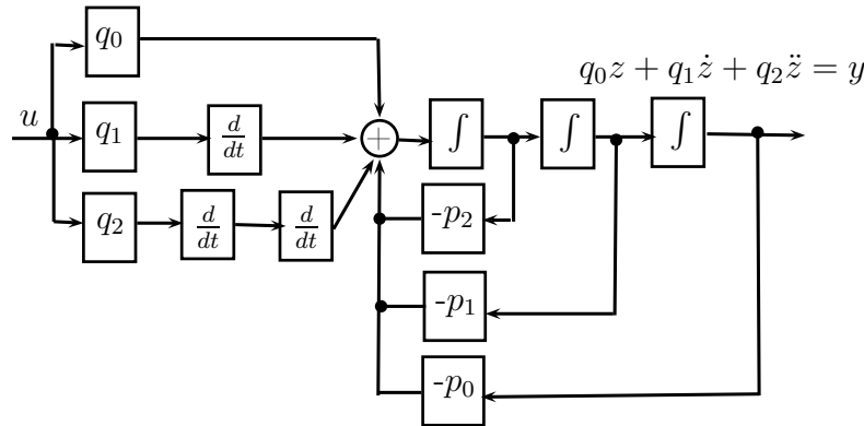
Gambar 7.7: Diagram superposisi.
