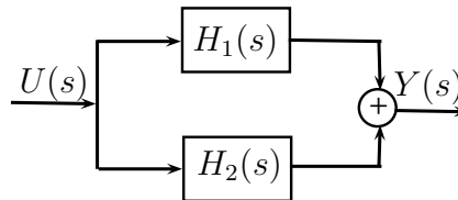
Gambar 7.2: Hubungan parallel dua sistem.
