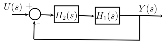
Gambar 7.14: Diagram Balok Umpan Balik plan H_1(s) dan kontroler H_2(s)
