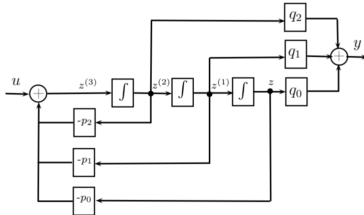
Gambar 7.5: Diagram realisasi.
