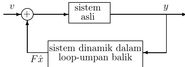
Gambar 5.6: Simbolik diagram.
