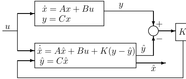
Gambar 5.2: Diagram alir sistem pengamat.
