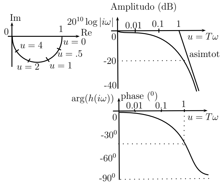
Gambar 7.12: Diagram Nyquist dan Bode.
