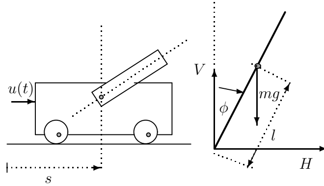
Gambar 2.2: Pendulum-terbalik.
