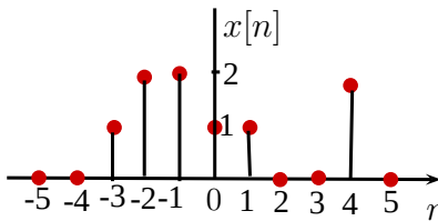
Gambar 8.2: Sistem Waktu Diskrit
