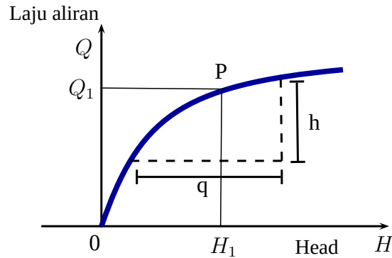
Gambar 2.7: Karakteristik Katup
