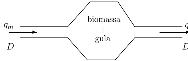
Gambar 2.5: Bioreaktor.
