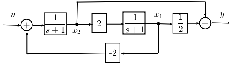
Gambar 7.11: Diagram Blok Dekomposisi h(s)
