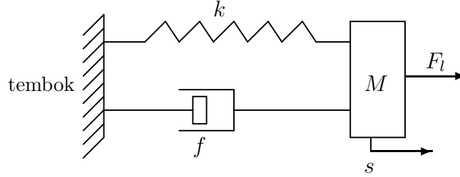
Gambar 2.4: Struktur Mekanika.
