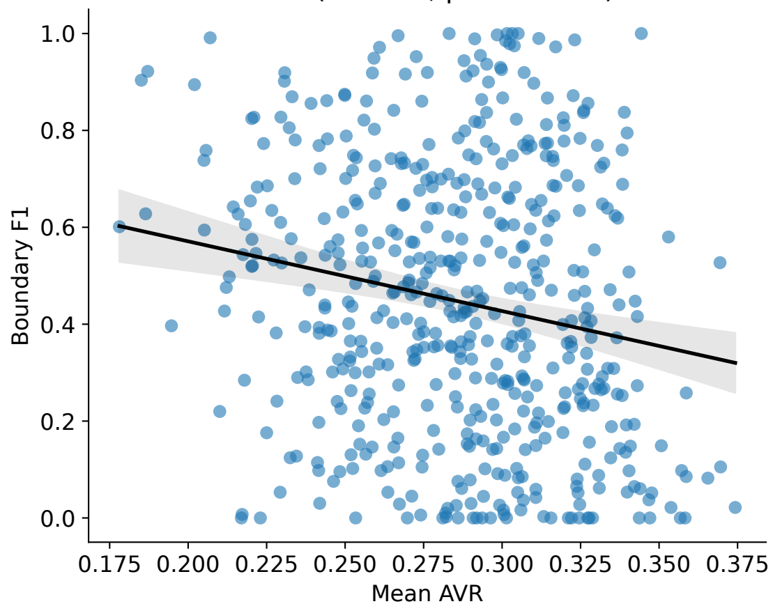
UNet ( r=-0.19 , p=1.62e-05 )
