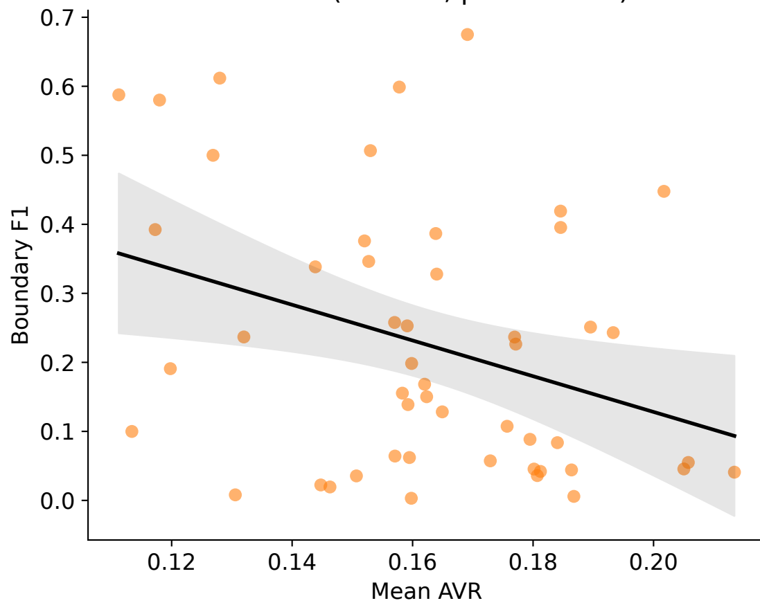
Mamba ( r=-0.34 , p=1.63e-02 )
