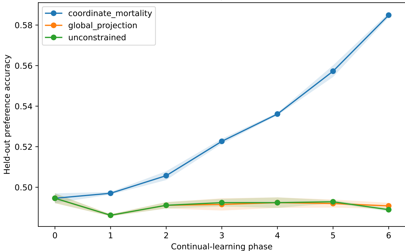
Qwen3-14B | benign shift
