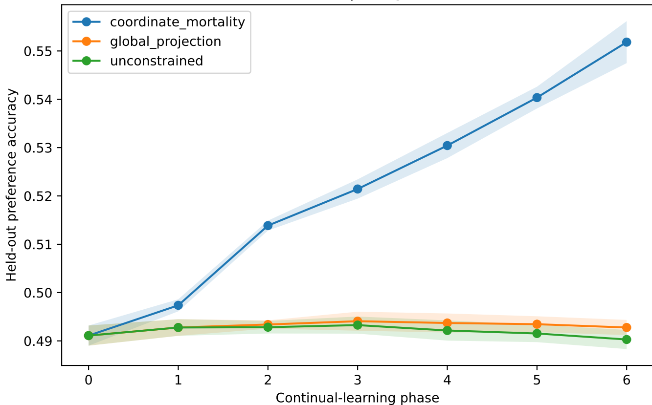
Qwen3-8B | benign shift
