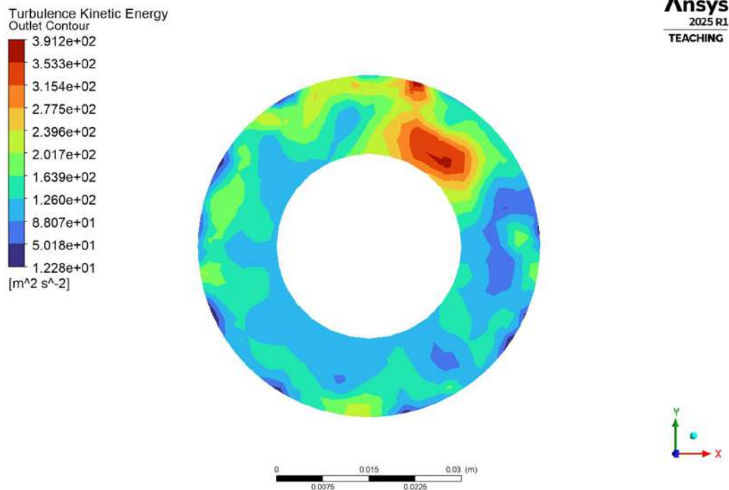
4.1.4.1(d) Outlet Turbulence Kinetic Energy
