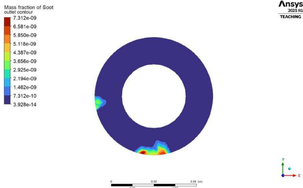
4.1.6.3(d) Outlet Soot mass fraction
