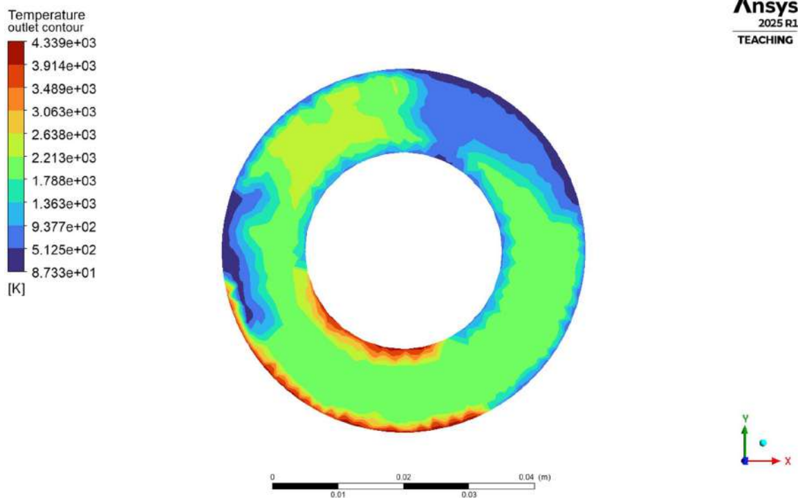
4.1.3.2(d) Outlet Temperature Contour
