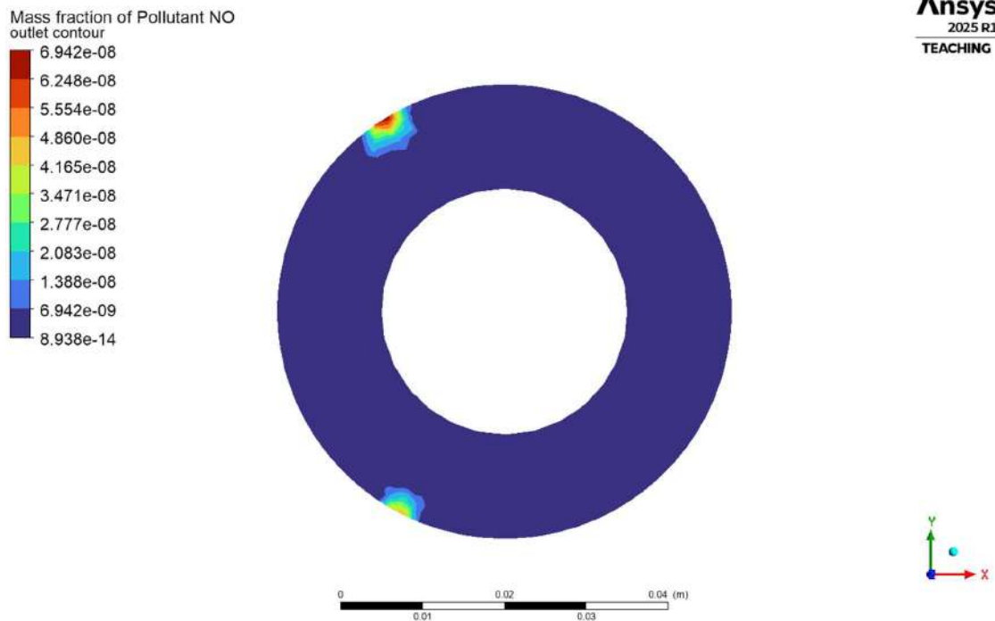
4.1.5.2(d) Outlet NO mass fraction
