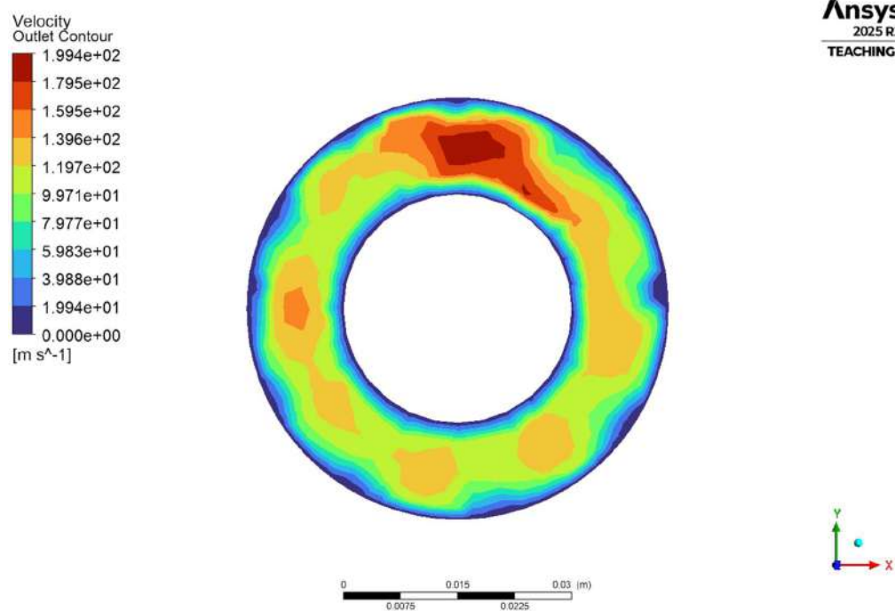
Fig.4.1.2.1(d) Outlet velocity Contour
