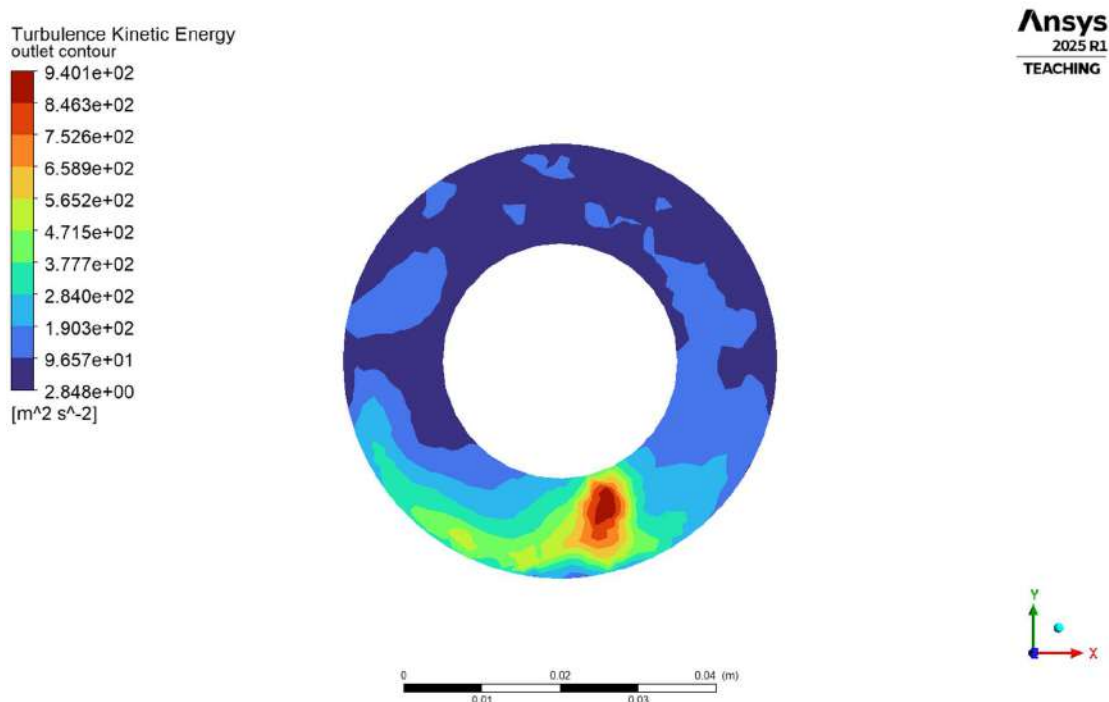
4.1.4.3(d) Outlet Turbulence Kinetic Energy
