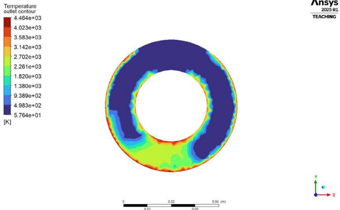
4.1.3.3(d) Outlet Temperature Distribution
