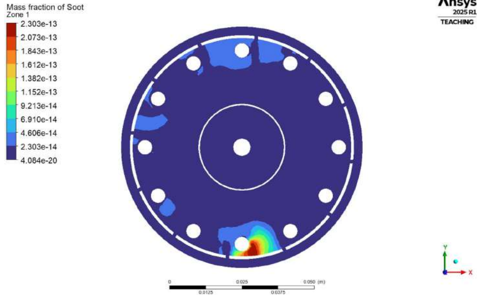
4.1.6.2(b) Zone 1 Soot mass fraction
