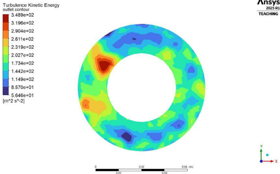
4.1.4.2(d) Outlet Turbulence Kinetic Energy
