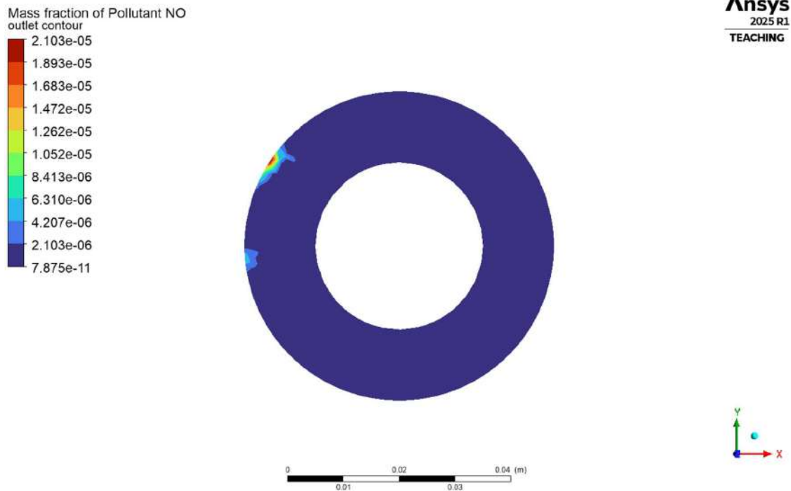
4.1.5.3(d) Outlet NO mass fraction
