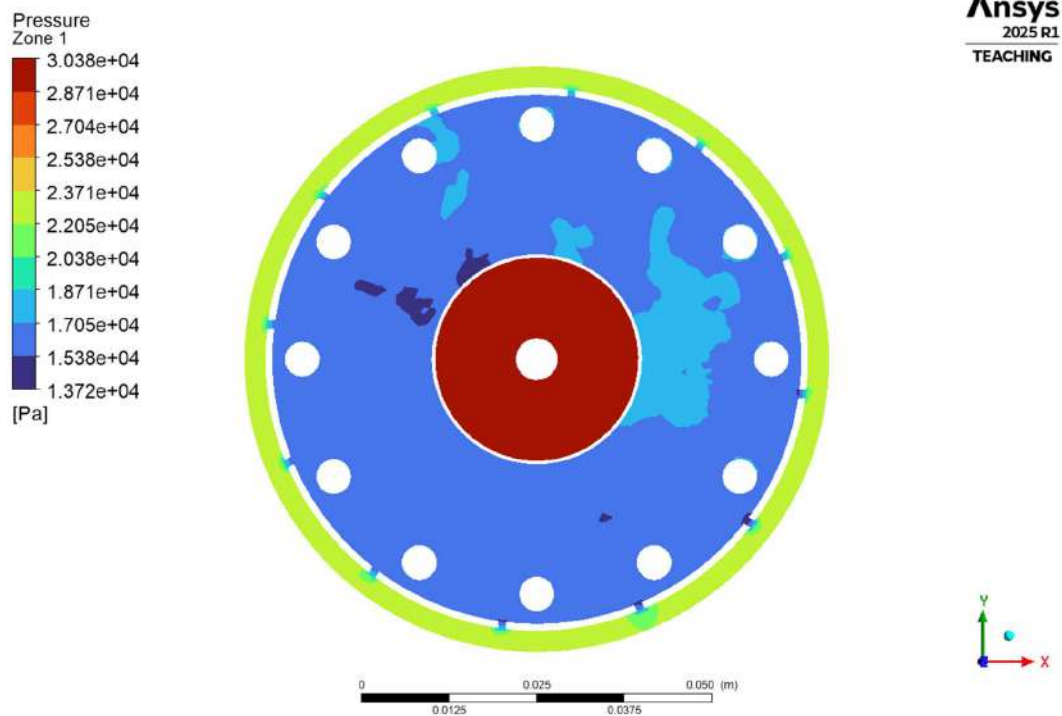
Fig.4.1.1.1(b) Zone 1 Pressure Contour.
