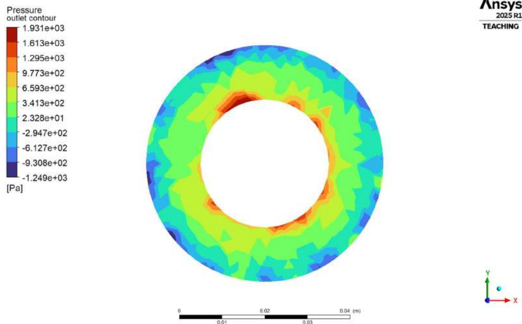
Fig.4.1.1.2(d) Outlet Pressure Contour.
