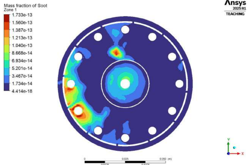
4.1.6.1(b) Zone 1 Soot mass fraction
