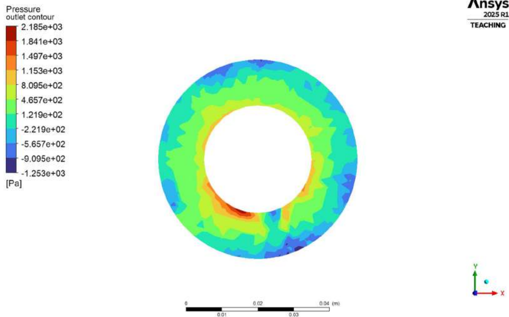
Fig.4.1.1.3(d) Outlet Pressure Contour.
