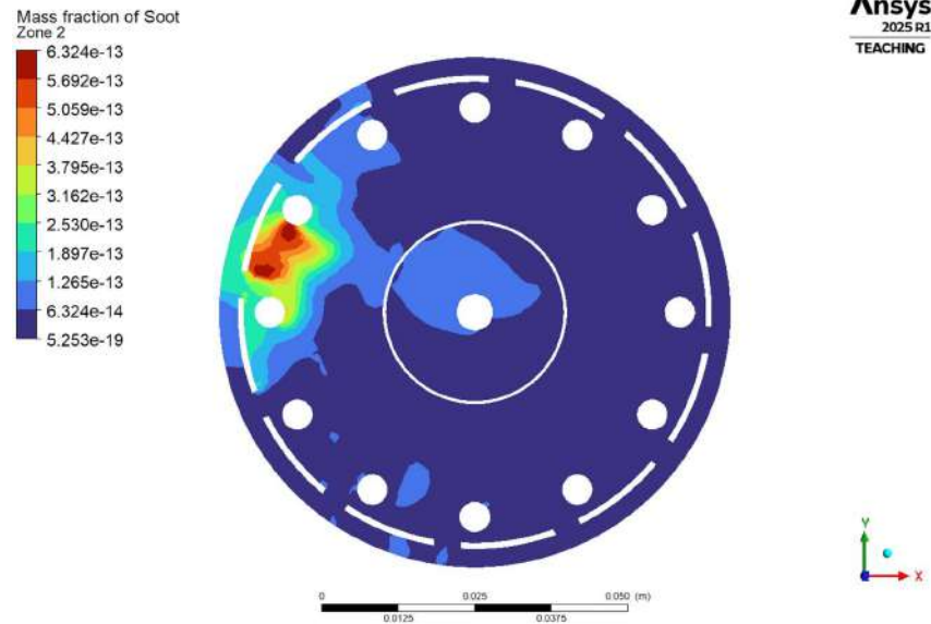
4.1.6.1(c) Zone 2 Soot mass fraction
