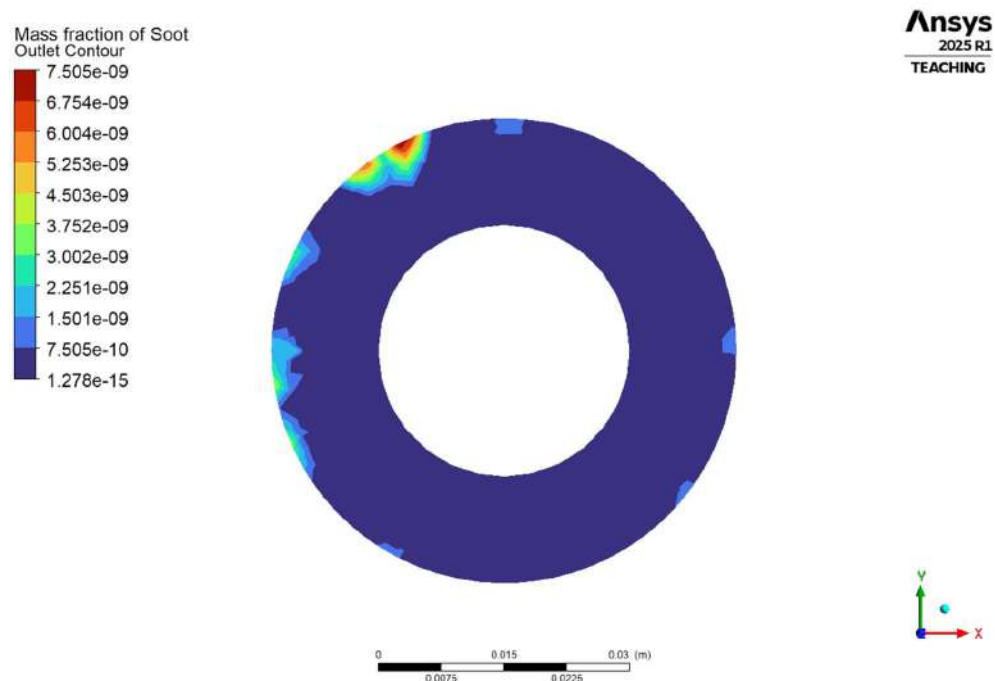
4.1.6.1(d) Outlet Soot mass fraction
