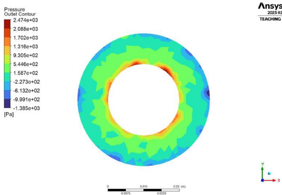
Fig.4.1.1.1(d) Outlet Pressure Contour.
