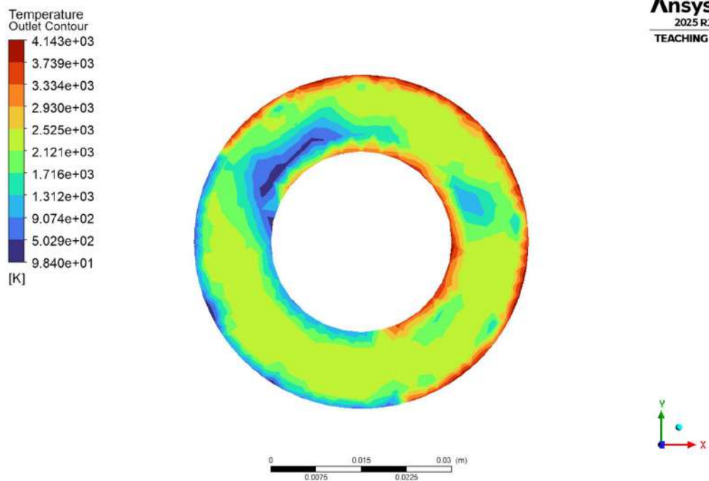
4.1.3.1(d) Outlet Temperature Contour
