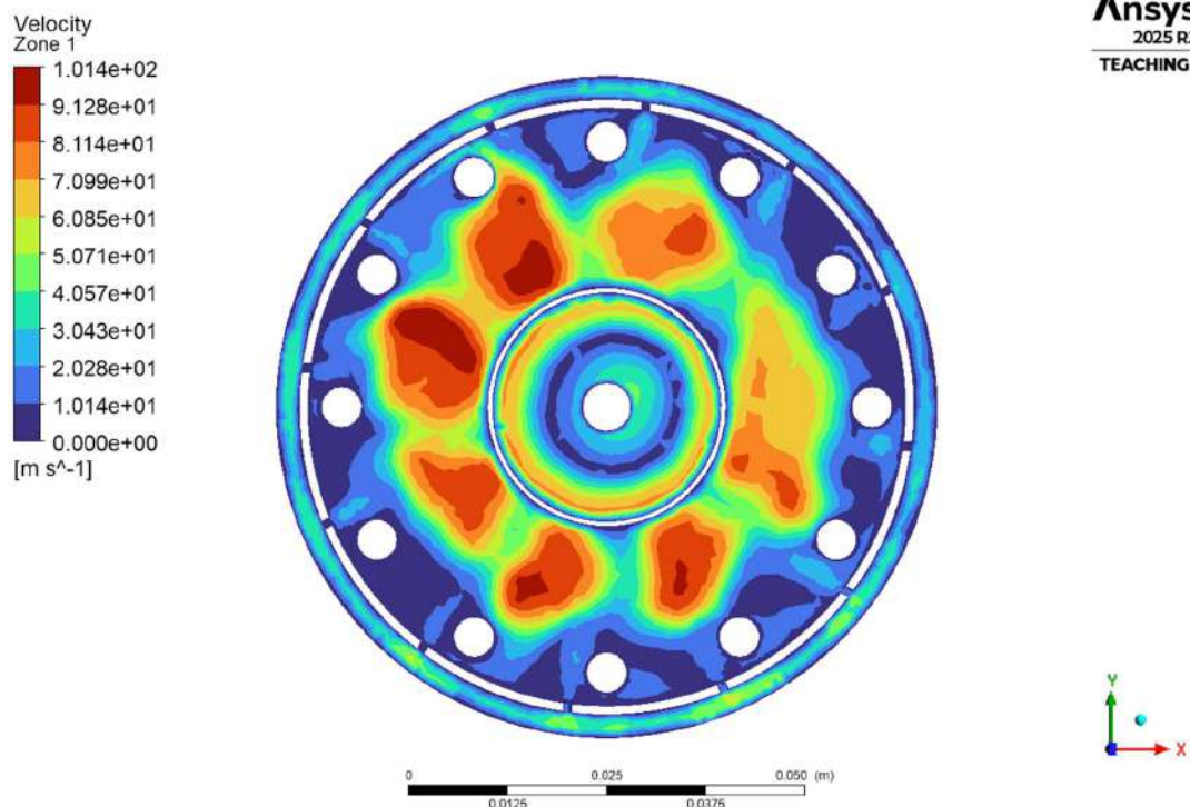
Fig.4.1.2.1(b) Zone 1 velocity Contour
