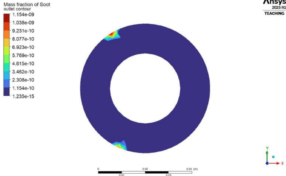
4.1.6.2(d) Outlet Soot mass fraction
