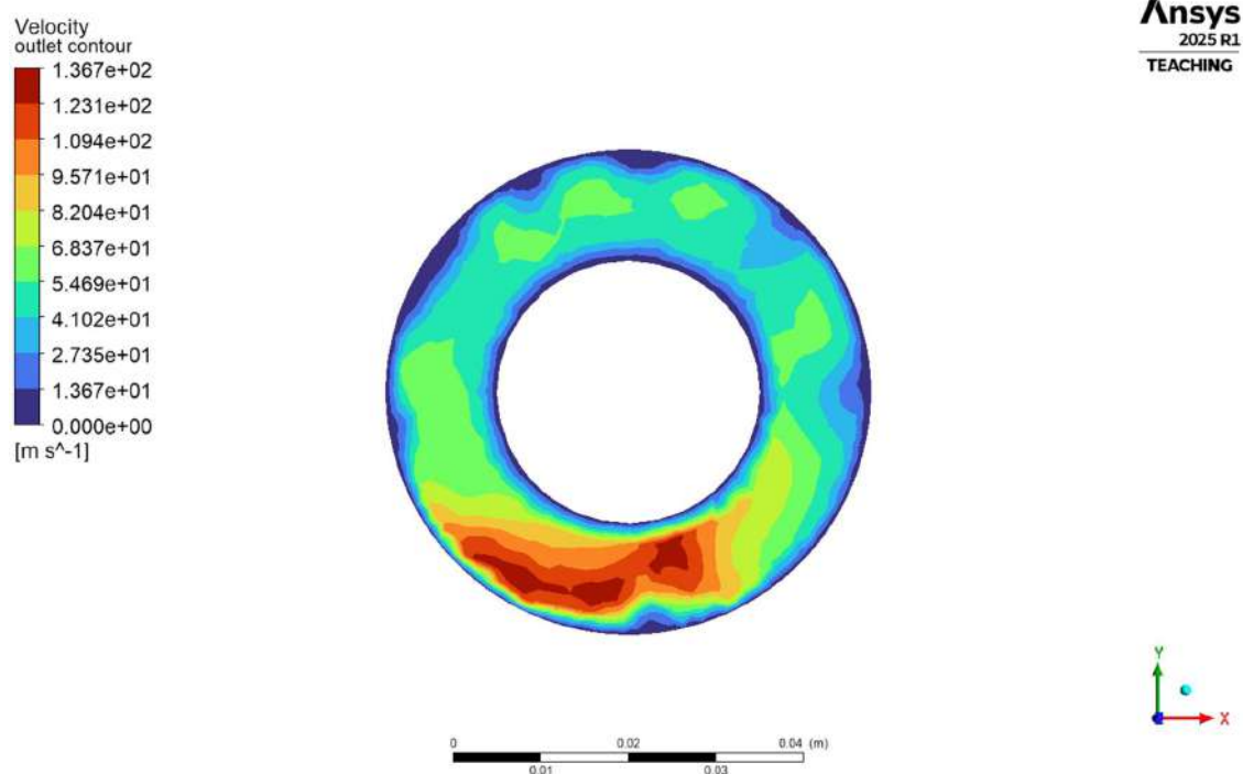
Fig.4.1.2.3(d) Outlet velocity Contour
