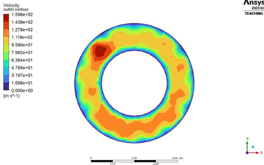
Fig.4.1.2.2(d) Outlet velocity Contour
