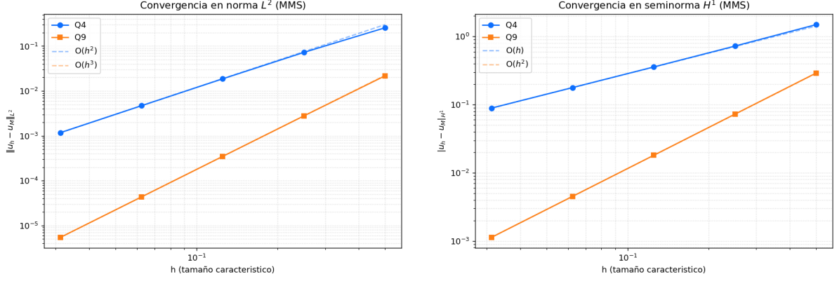
(a) Norma L^2 del desplazamiento.
