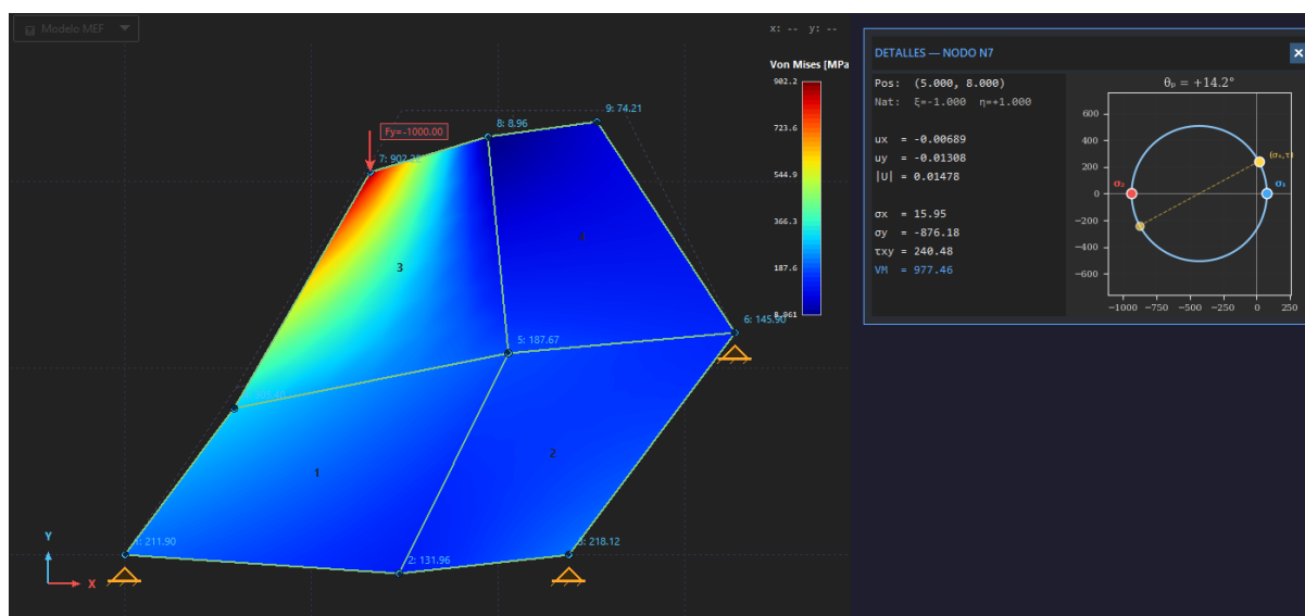
Figura 2.5 Visualización de resultados en el post-proceso.
