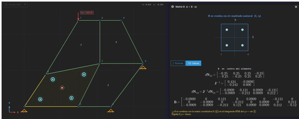
Figura B.9: Módulo M3 (matriz de deformación B ). La cadena de derivadas \partial N_{\xi\eta} \rightarrow J^{-1} \rightarrow B evaluada en el punto natural, anclada a los puntos de Gauss del elemento.
