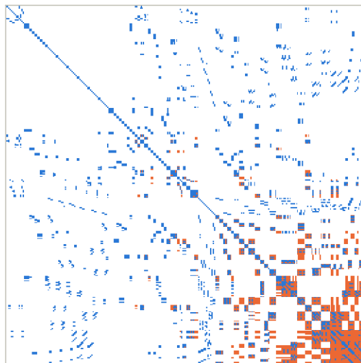
L + U : 27 104 coeficientes ( 1,7 \times \text{nnz}(K_{ff}) )
