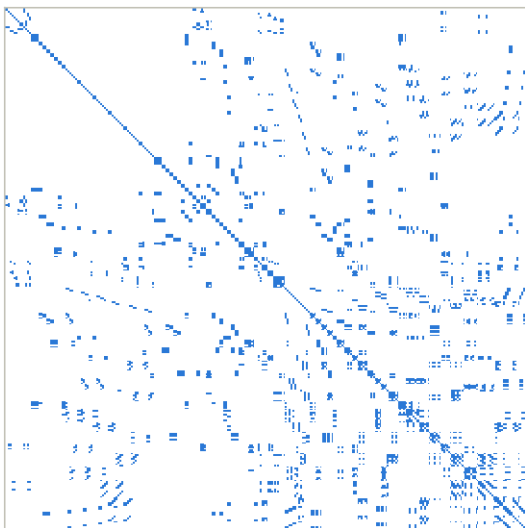
K_{ff} , reordenada con MMD_AT_PLUS_A 15 600 no nulos
