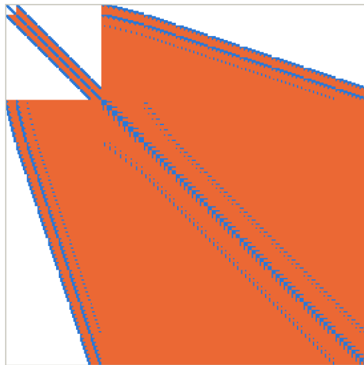
L + U : 232 880 coeficientes ( 14,9 \times \text{nnz}(K_{ff}) )
