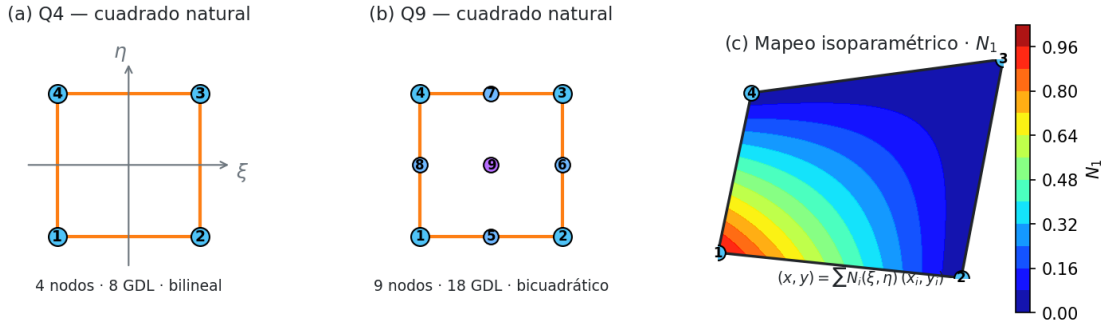
Figura 1.1: Elementos isoparamétricos Q4 y Q9 y el mapeo isoparamétrico al espacio físico.
