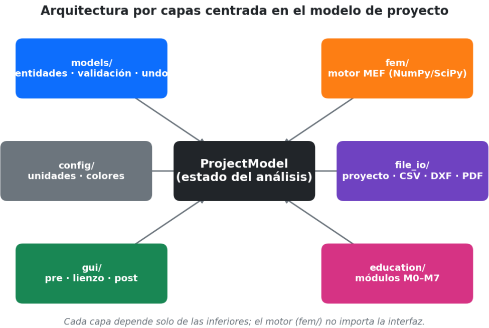
Figura 2.1: Arquitectura por capas centrada en el modelo de proyecto.
