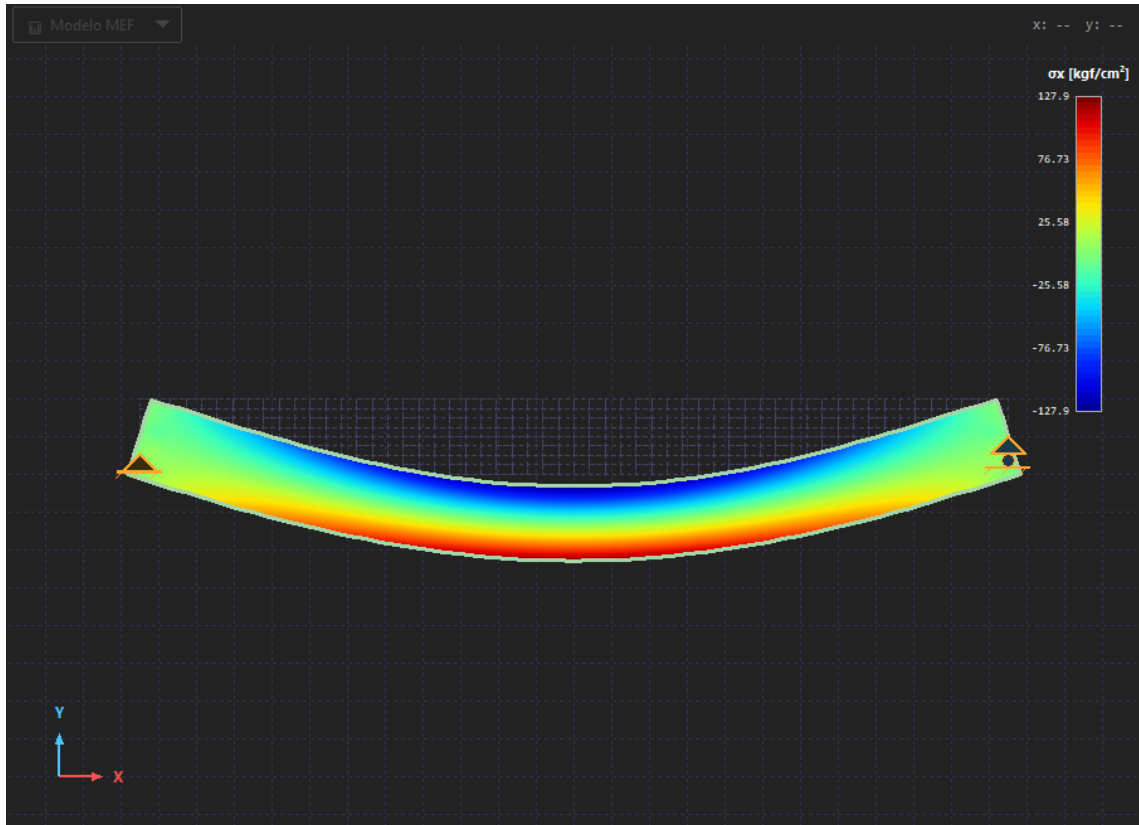
Figura 3.2: Post-proceso de EduFEM: campo de tensión normal \sigma_x sobre la configuración deformada de la viga de Timoshenko ( 56 \times 8 Q9). La gradación lineal de \sigma_x en el peralte –tracción (rojo) en la fibra inferior, compresión (azul) en la superior y eje neutro (verde)– coincide con la predicción de la teoría de vigas.
