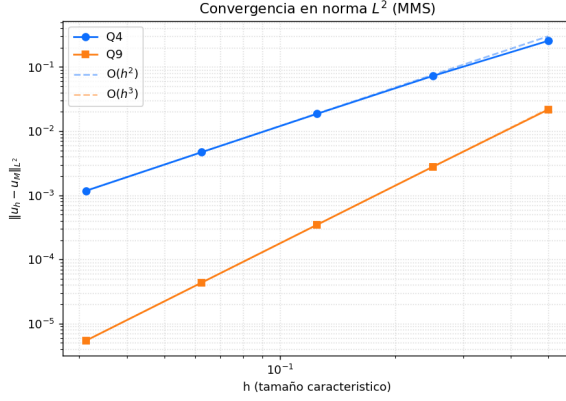
(a) Norma L^2 del desplazamiento.
