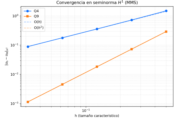
(b) Seminorma H^1 del desplazamiento.
